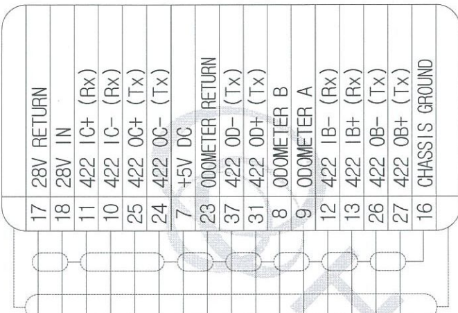
P4(진북기준기)
