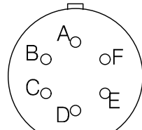
YH3474W10-6P 연결기 후면도 #20-6EA
