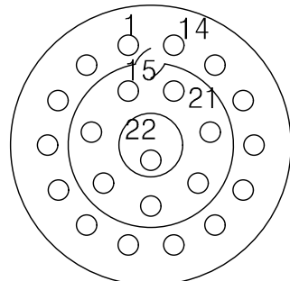
MS27474T12B35P 연결기 후면도 #22D-22EA
