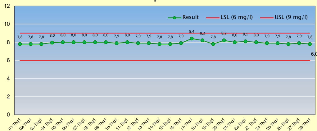
pH
