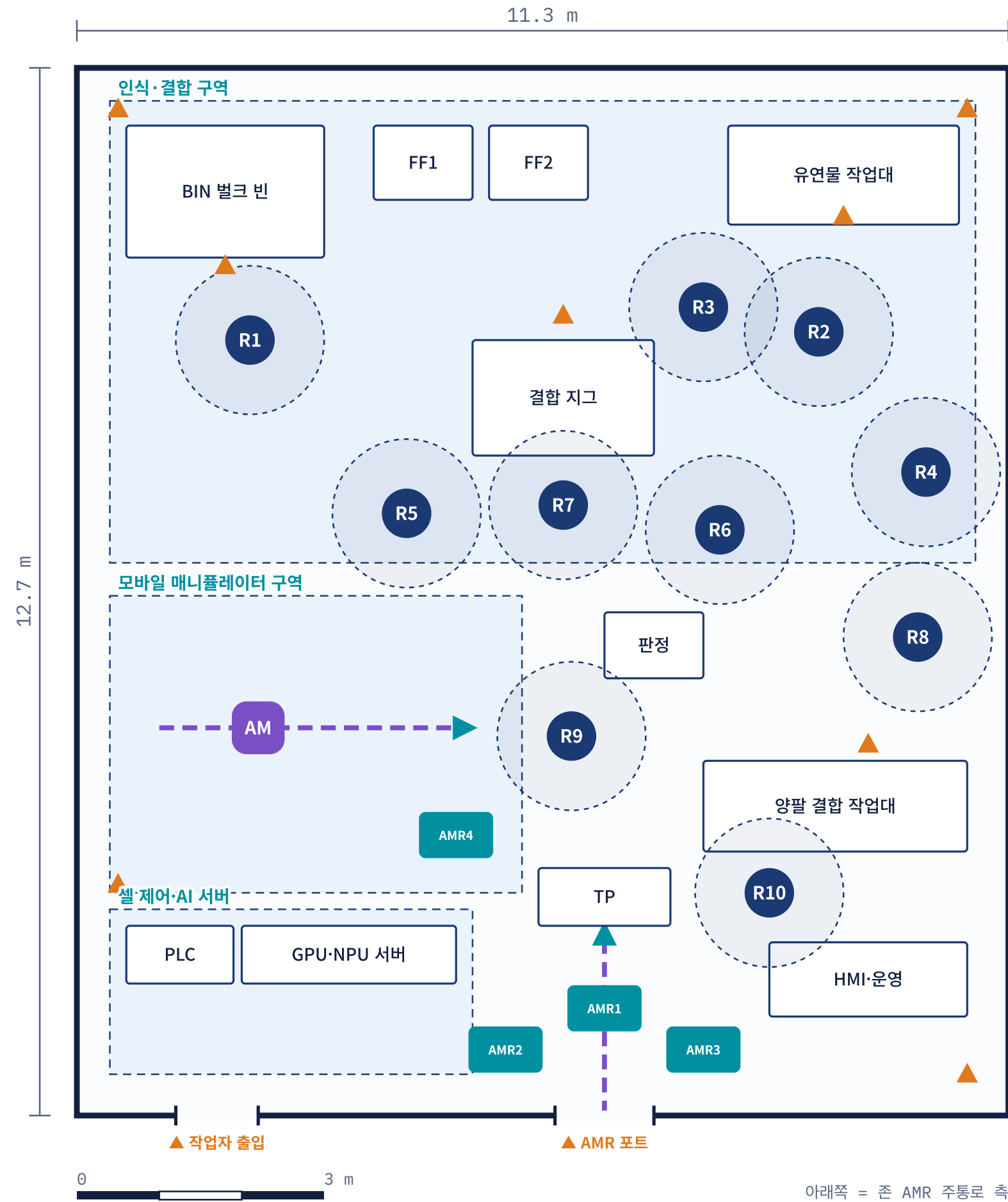
A-3-1 개념 배치도 (설계 추정 · 실측 전) — 아래쪽이 존 주통로
