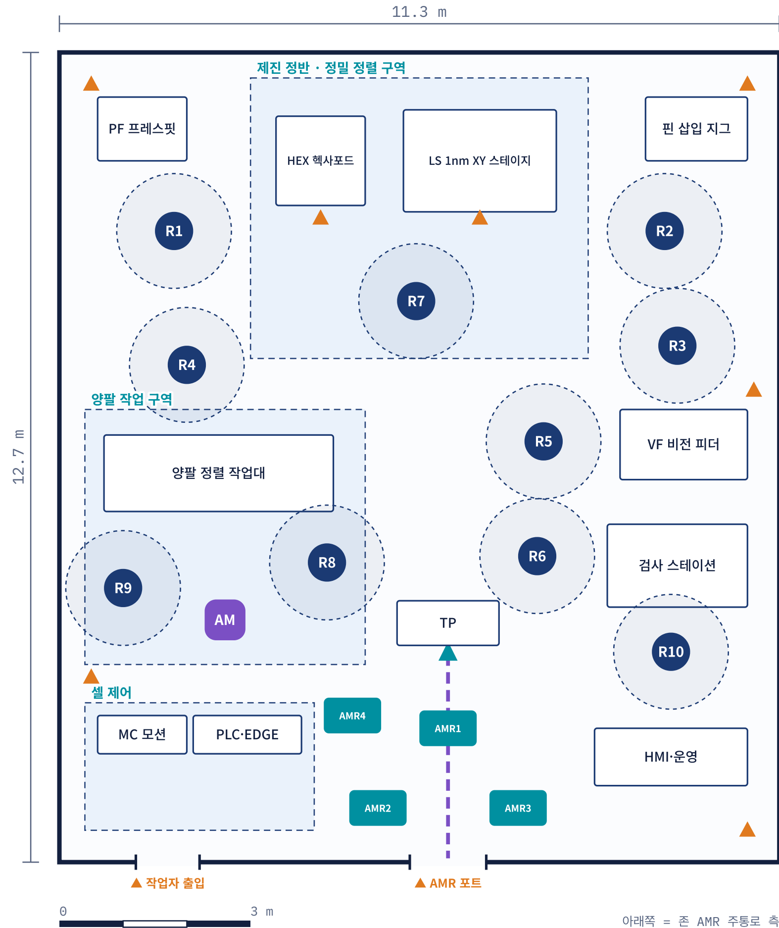
A-3-3 개념 배치도 (설계 추정 · 실측 전) — 아래쪽이 존 주통로
