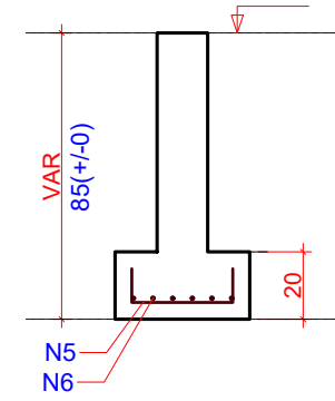
3 DETALHAMENTO SAPATA E PILAR ESCALA 1:25
