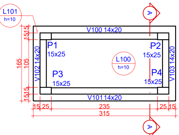
4 PLANTA DE FORMAS - TOPO ESCALA 1:50
