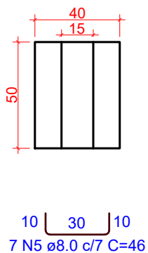
3 DETALHAMENTO SAPATA E PILAR ESCALA 1:25
