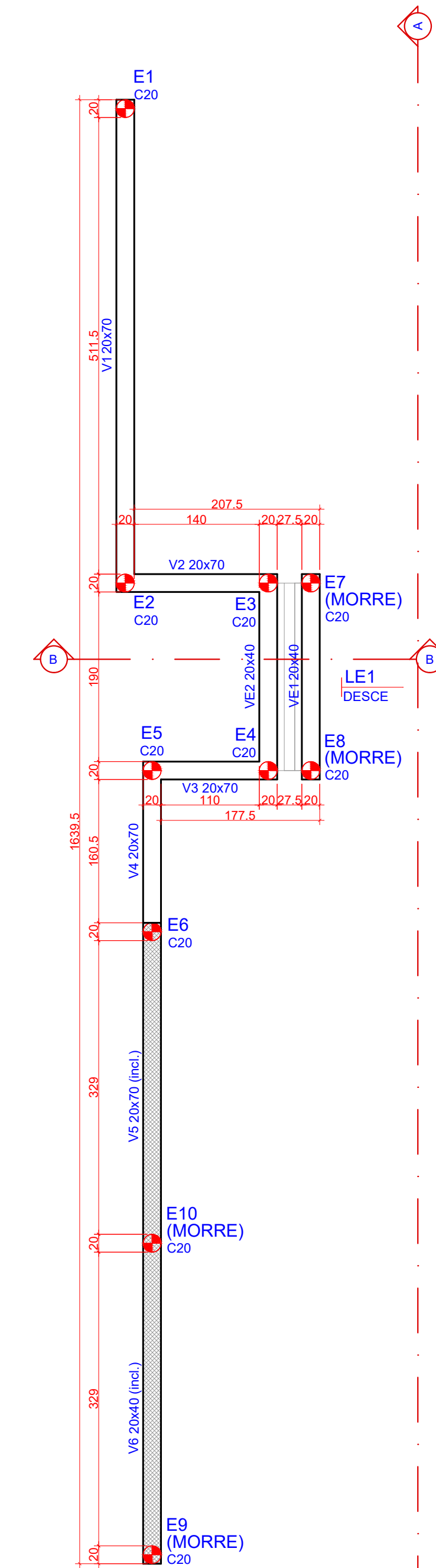
1 PLANTA DE FORMAS ESCALA 1:50
