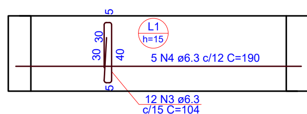
4 ARMAÇÃO POSITIVA DA LAJE ESCALA 1:25
