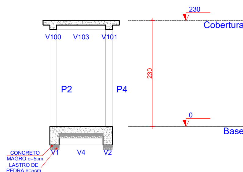
5 CORTE A-A ESCALA 1:50
