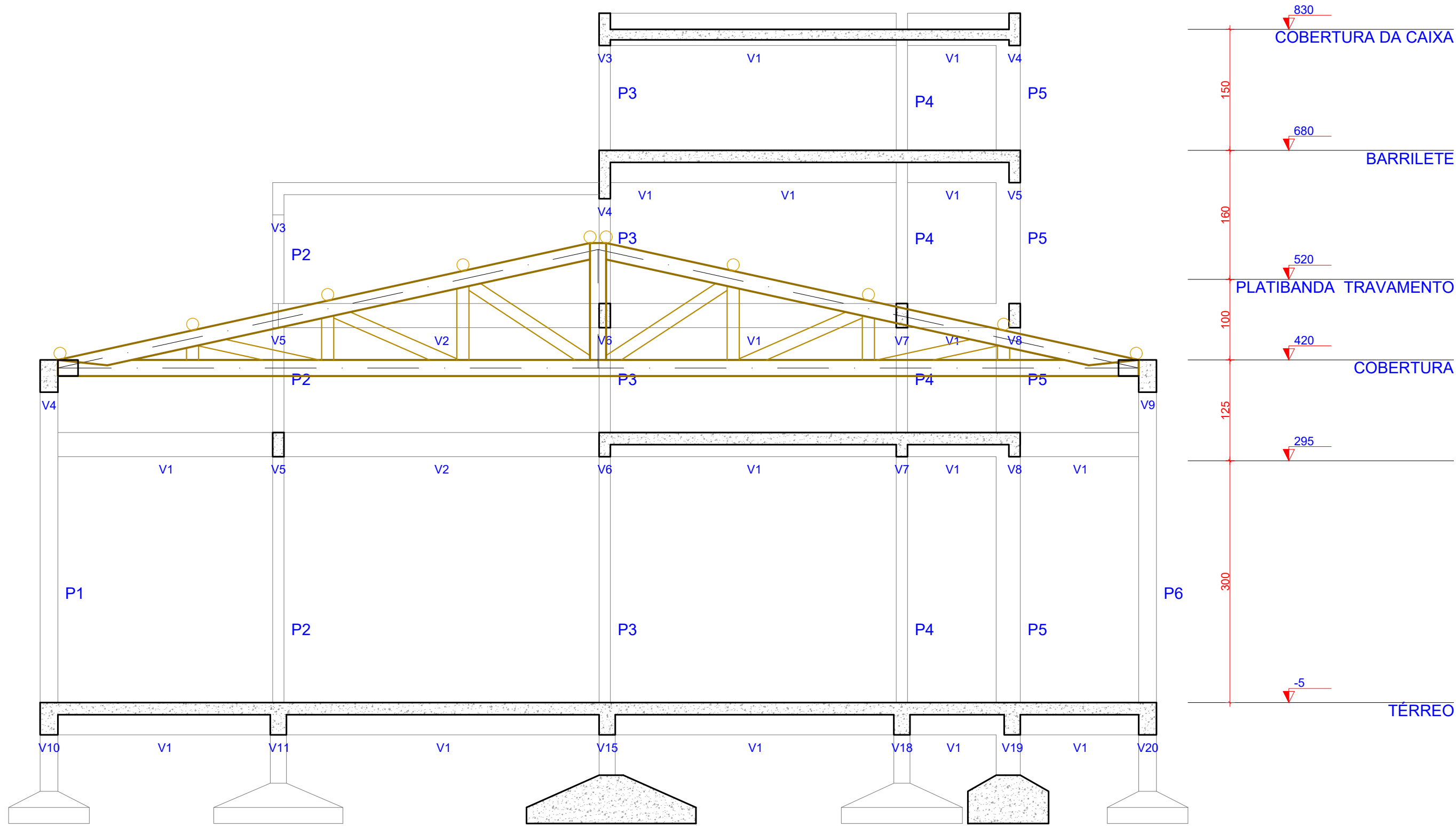
1 CORTE C-C ESCALA 1:50
