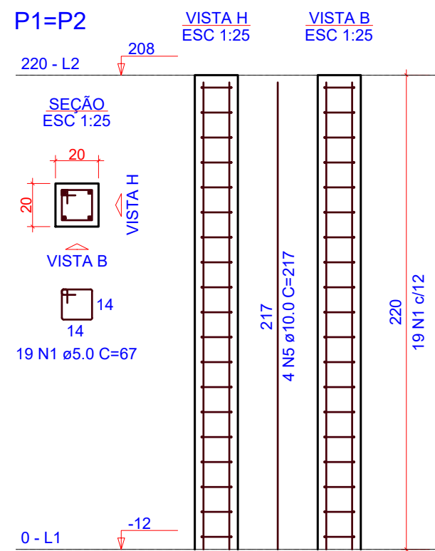
5 DETALHAMENTO PILARES ESCALA 1:25
