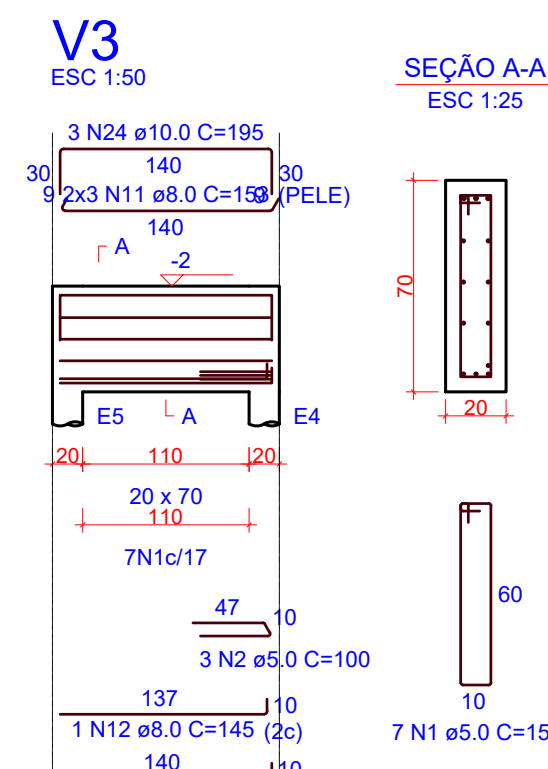
SEÇÃO A-A ESC 1:25
