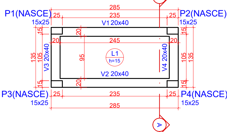
2 PLANTA DE FORMAS - BASE ESCALA 1:50
