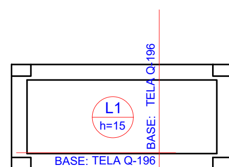
8 ARMAÇÃO POSITIVA DAS LAJES - BASE ESCALA 1:50
