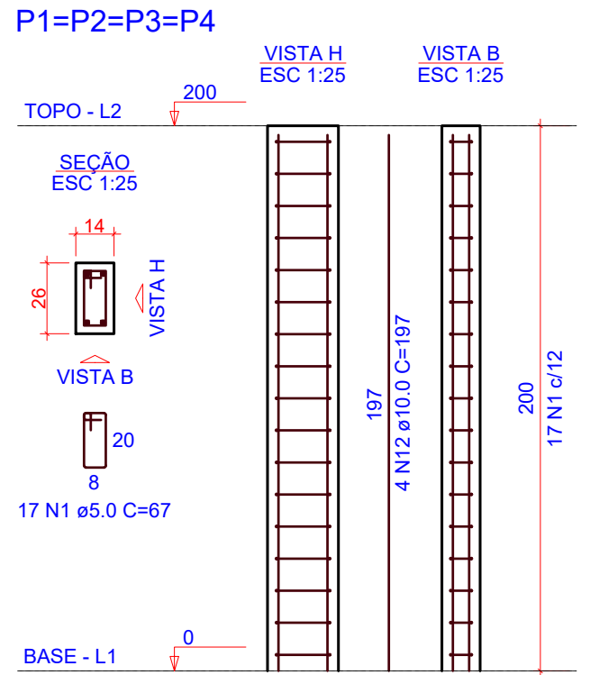
3 DETALHAMENTO PILARES ESCALA 1:25
