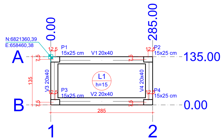
1 PLANTA DE LOCAÇÃO ESCALA 1:50
