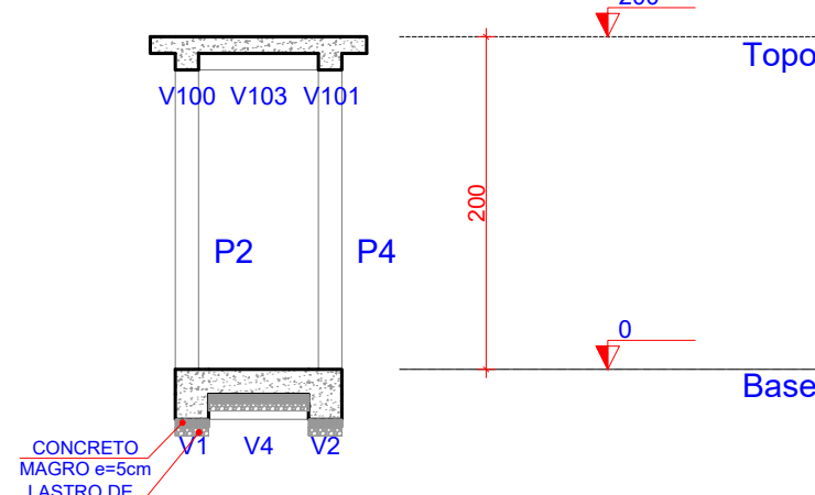
5 CORTE A-A ESCALA 1:50
