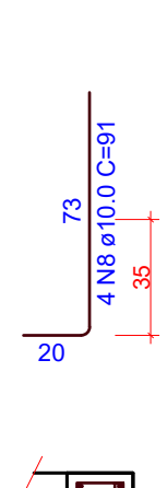
ESPERA P2 ESC 1:25
