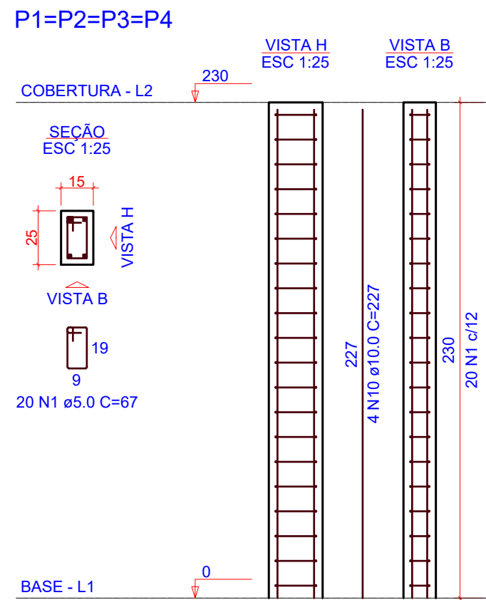
3 DETALHAMENTO PILARES ESCALA 1:25
