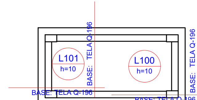
9 ARMAÇÃO POSITIVA DAS LAJES - TOPO ESCALA 1:50
