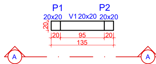
2 PLANTA DE FORMAS - TOPO ESCALA 1:50
