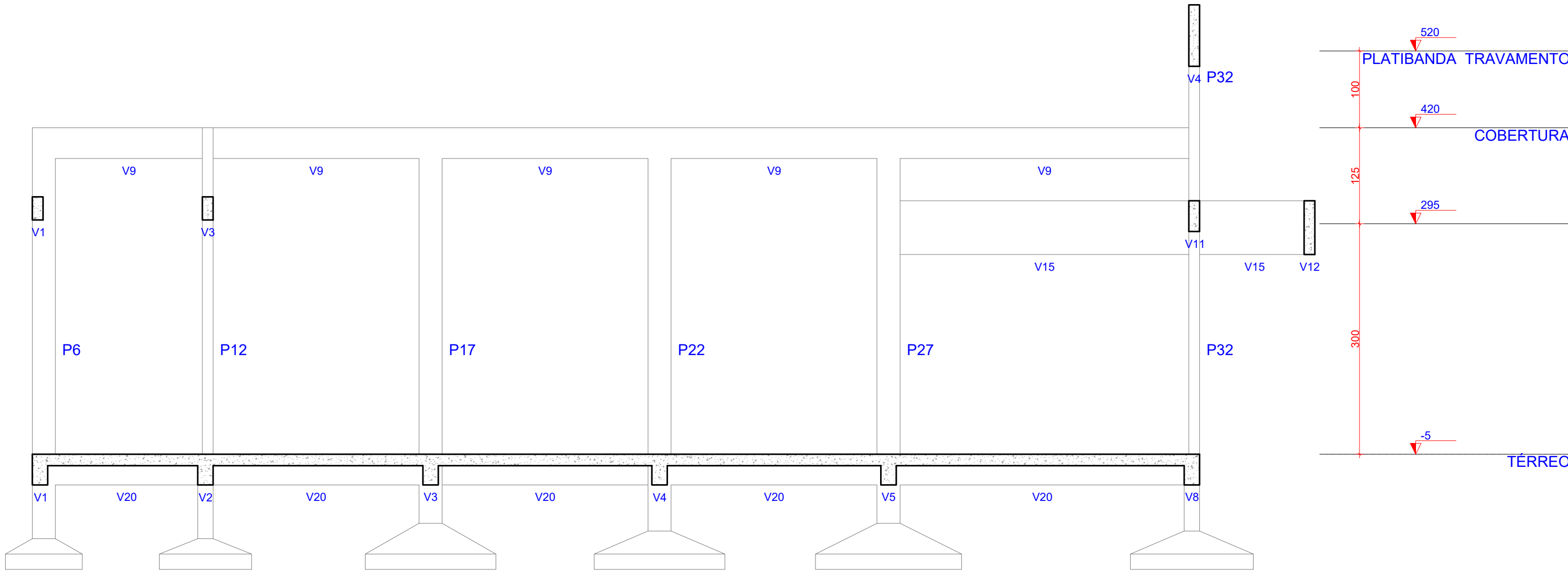
2 CORTE B-B ESCALA 1:50
