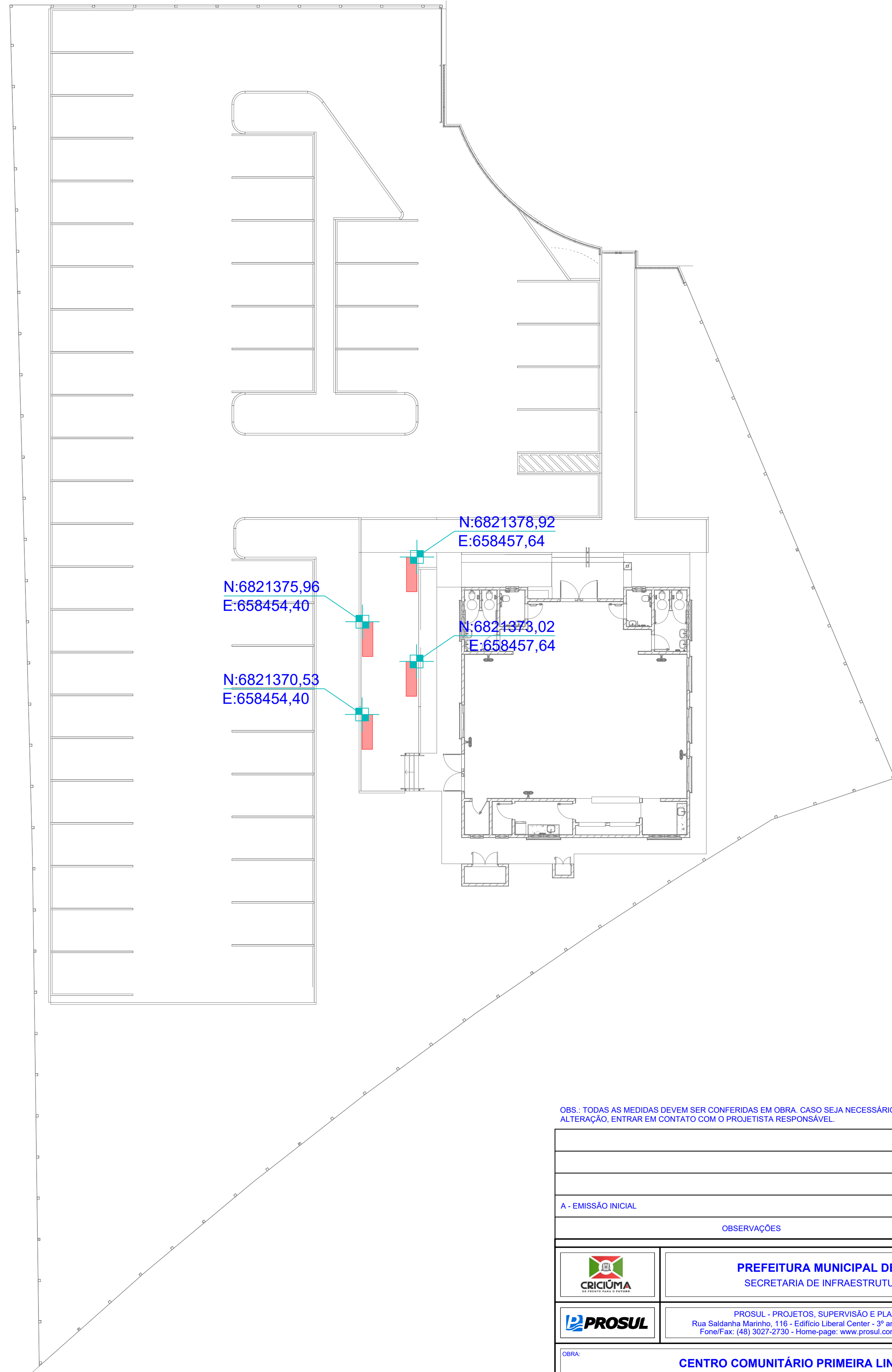
7 PLANTA SETORIZAÇÃO ESCALA REPRESENTATIVA
