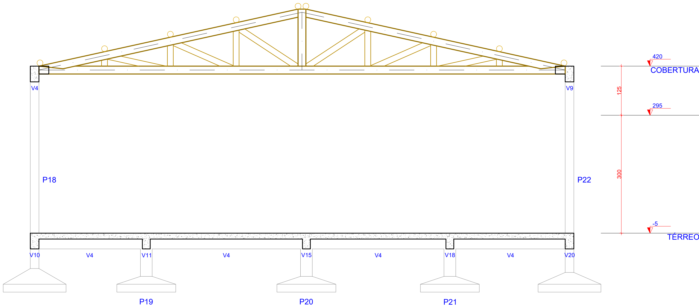
1 CORTE A-A ESCALA 1:50
