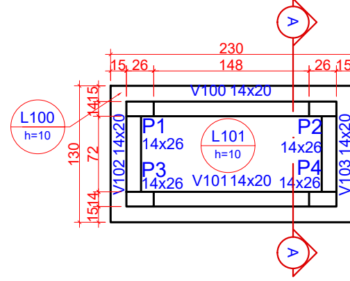
4 PLANTA DE FORMAS - TOPO ESCALA 1:50
