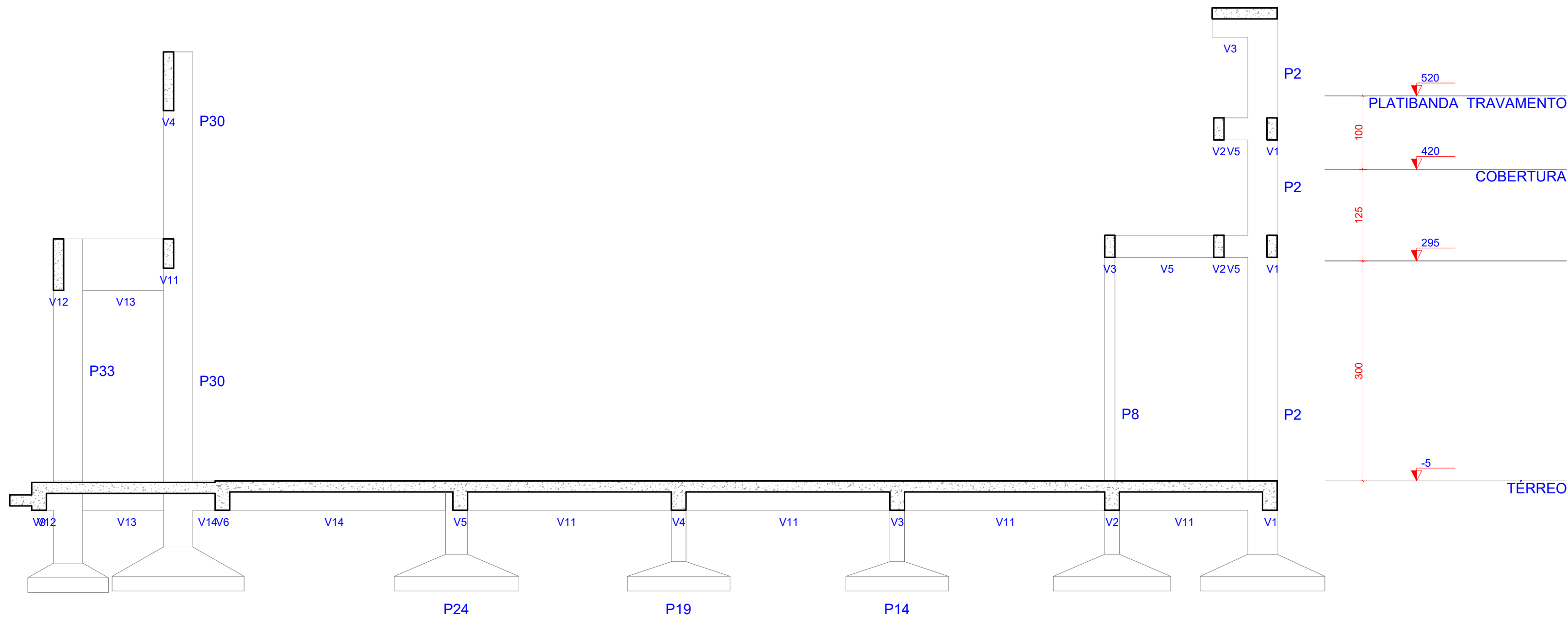
2 CORTE D-D ESCALA 1:50
