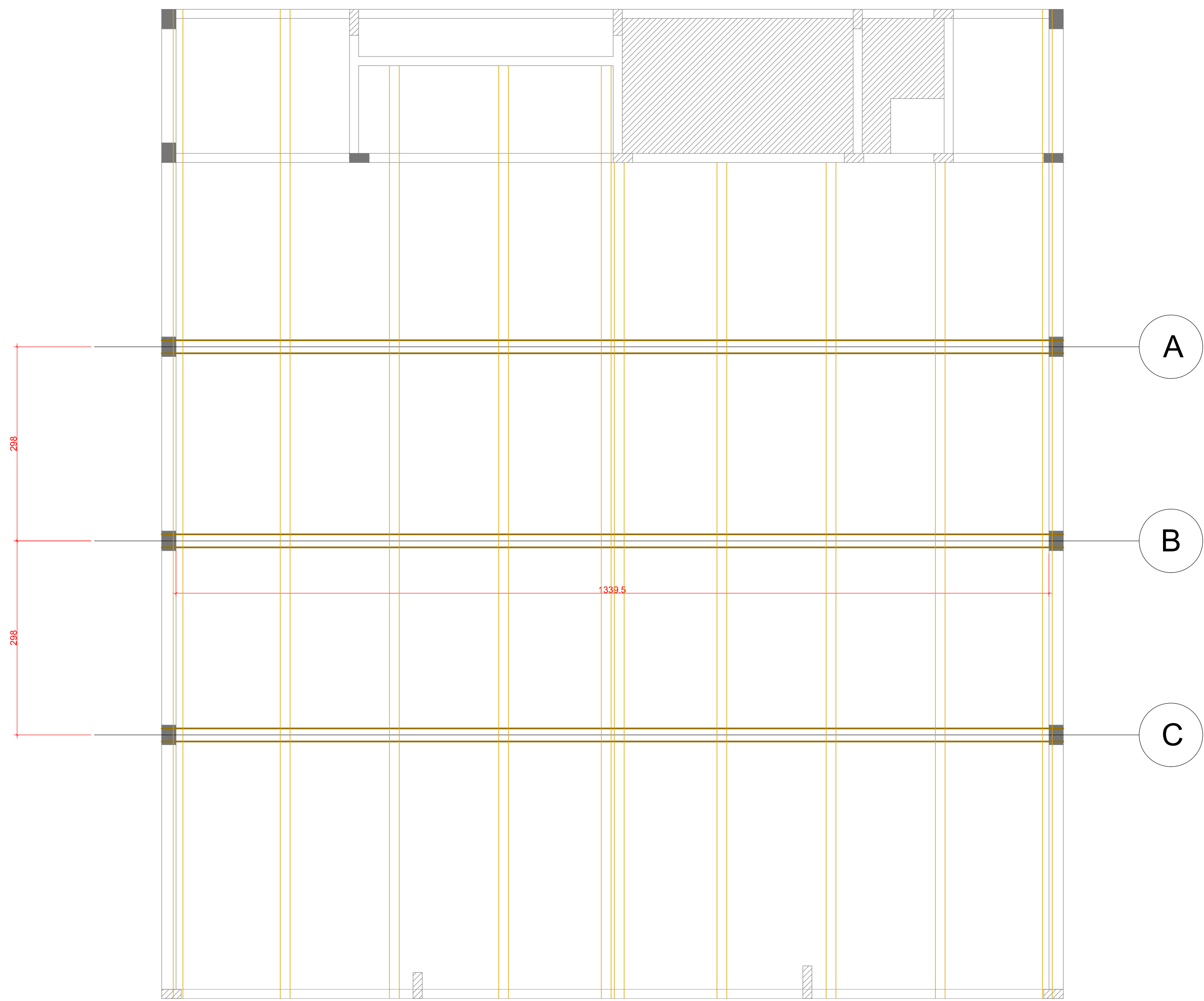
1 PLANTA DE FORMAS - COBERTURA (NÍVEL 420) ESCALA 1:50
