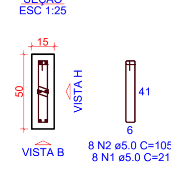
3 DETALHAMENTO SAPATA E PILAR ESCALA 1:25
