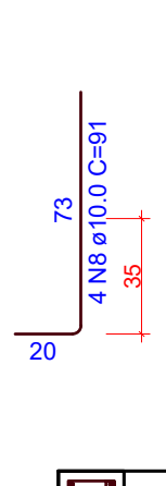
ESPERA P1 ESC 1:25
