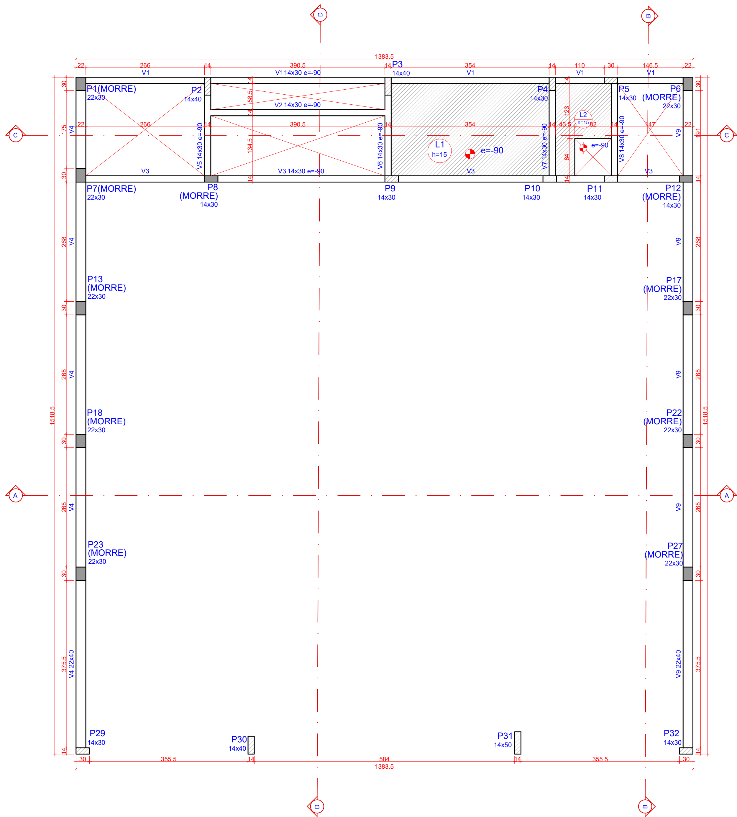
1 PLANTA DE FORMAS - COBERTURA (NÍVEL 420) ESCALA 1:50
