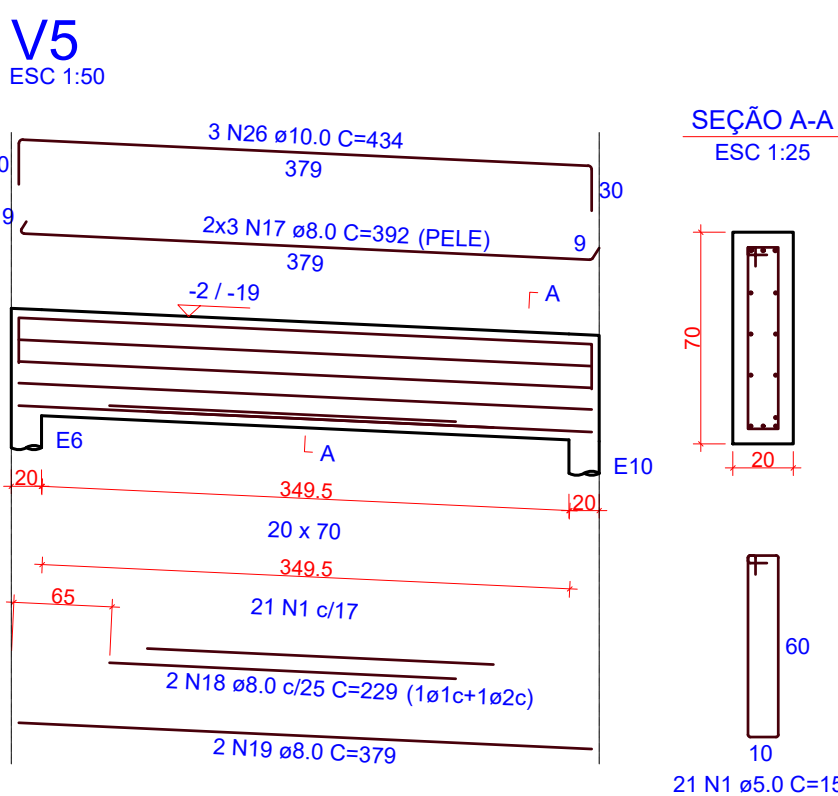
4 DETALHAMENTO VIGAS ESCALA INDICADA
