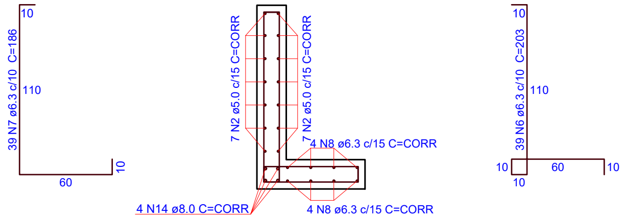
6 PLANTA DE ARMADURAS - DETALHE MURO M2 ESCALA 1:25
