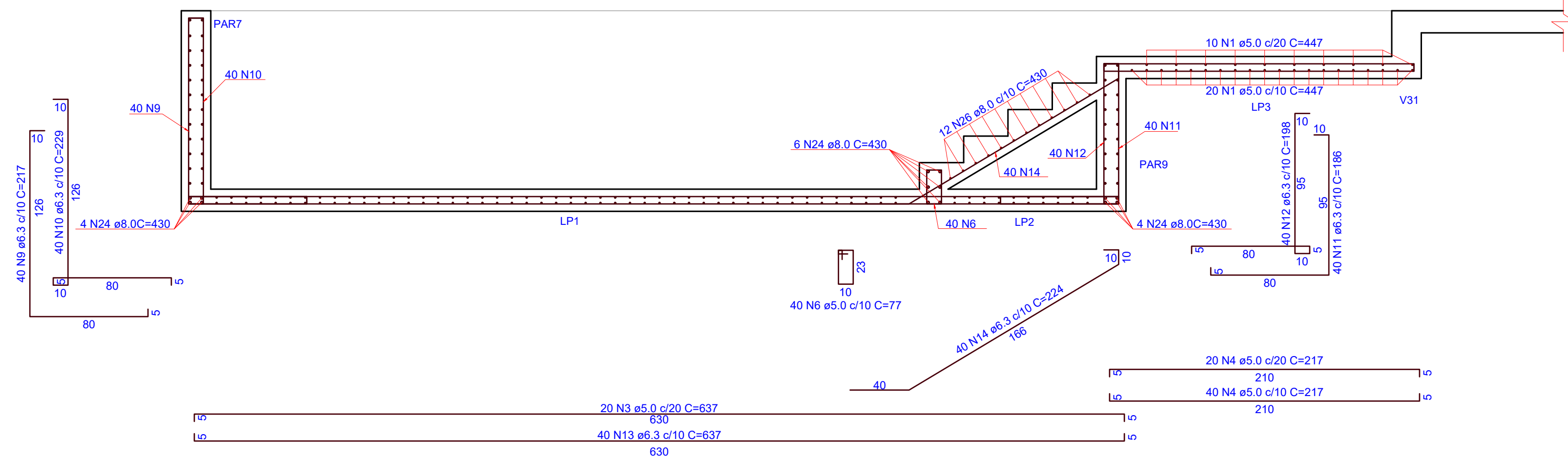
2 PLANTA DE ARMADURAS: CORTE F-F ESCALA 1:25
