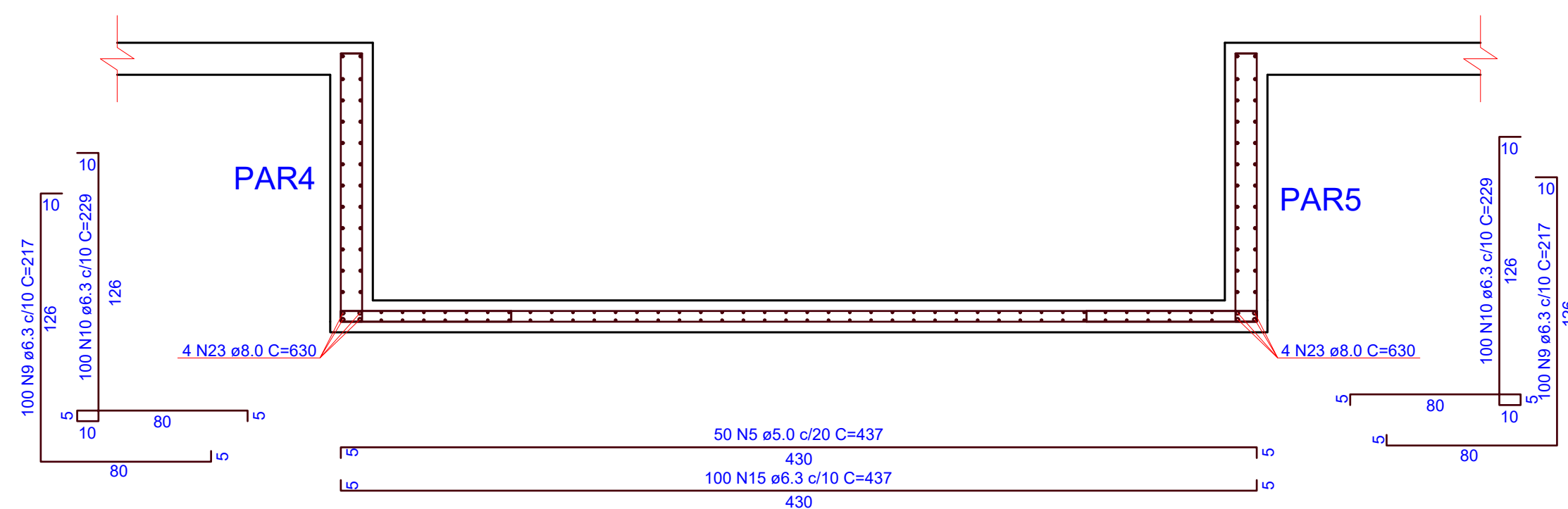
3 PLANTA DE ARMADURAS: CORTE G-G
