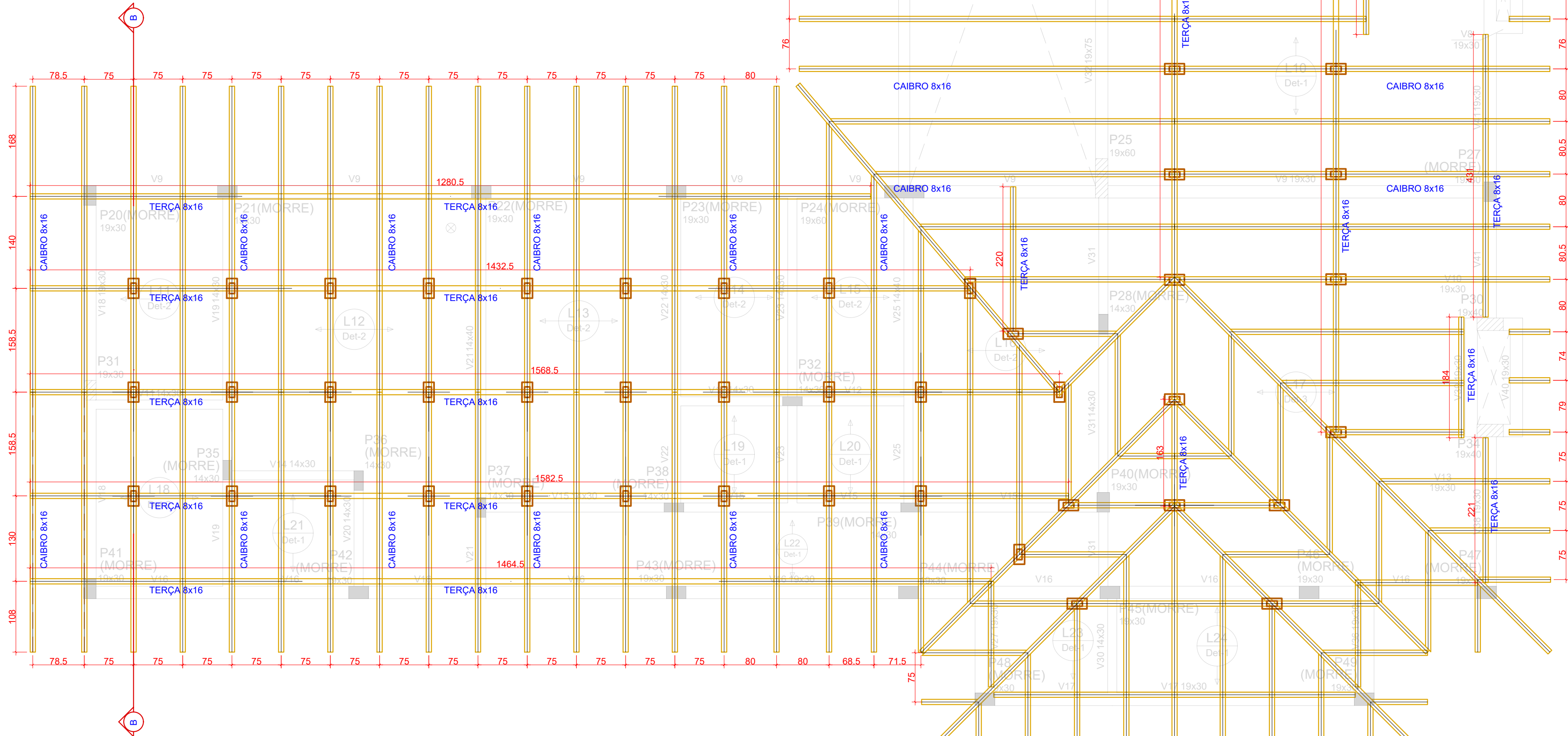
1 PLANTA BAIXA - COBERTURA MADEIRA ESCALA 1:50
