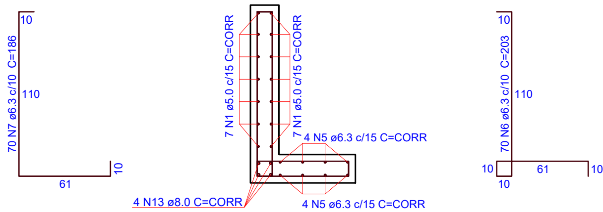
5 PLANTA DE ARMADURAS - DETALHE MURO M1 ESCALA 1:25
