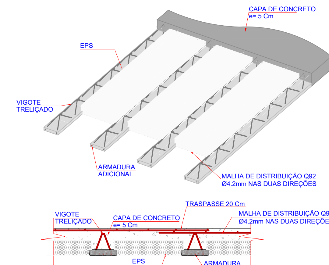
2 DETALHE 01 LAJE PRÉ-FABRICADA - TRELIÇADA ESCALA 1:20
