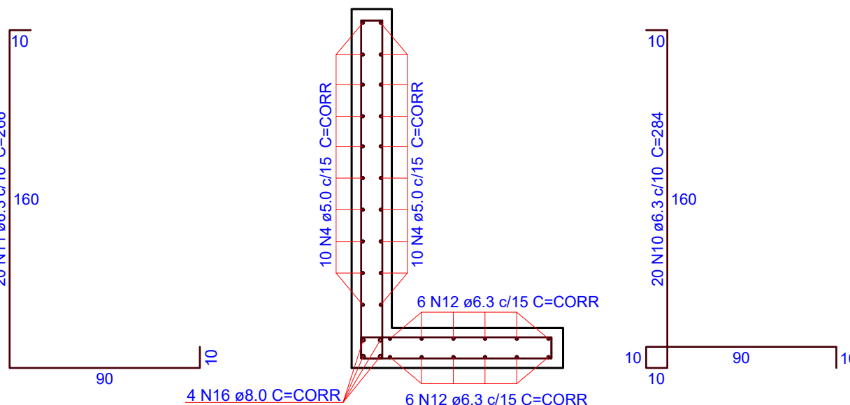
8 PLANTA DE ARMADURAS - DETALHE MURO M4 ESCALA 1:25
