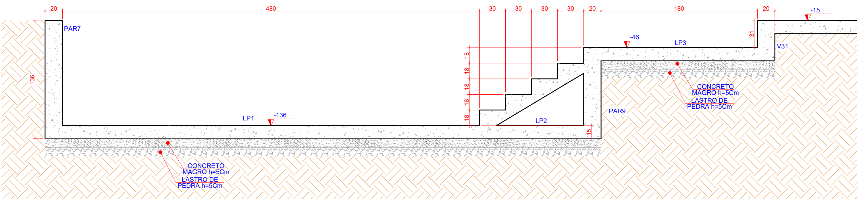
2 PLANTA DE FORMAS: CORTE F-F
