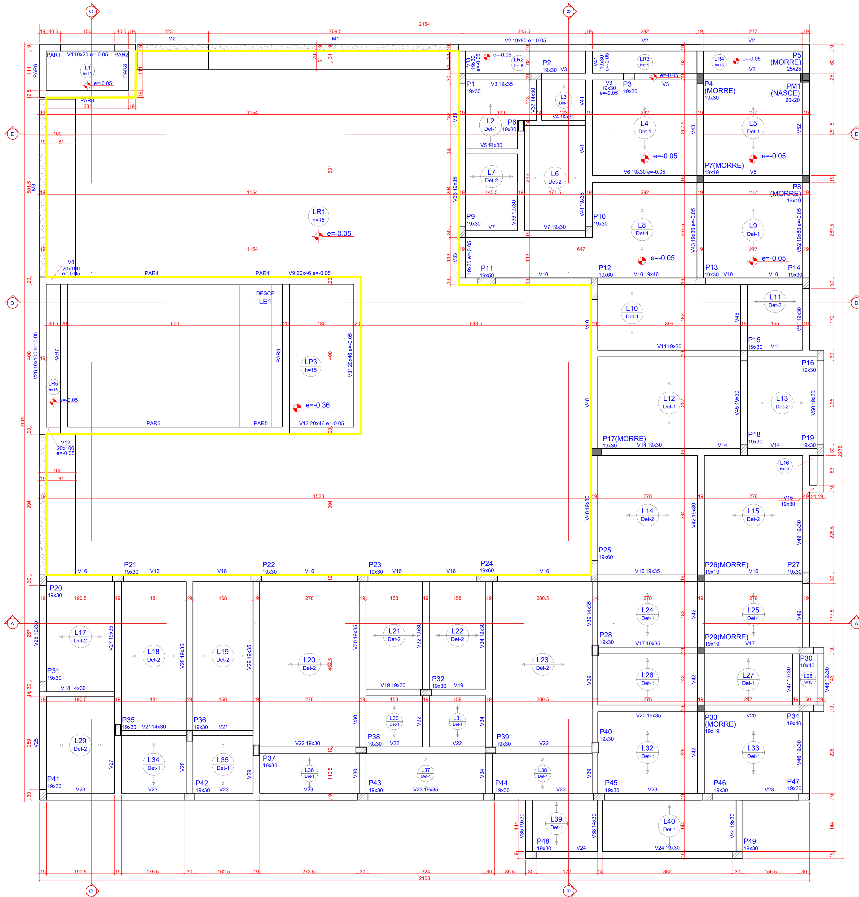
1 PLANTA DE FORMAS - TÉRREO (NÍVEL -0.10) ESCALA 1:50
