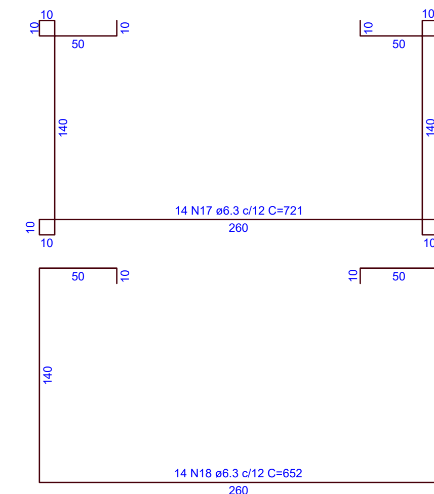
4 PLANTA DE ARMADURAS: PLANTA BAIXA CASA DE MÁQUINAS
