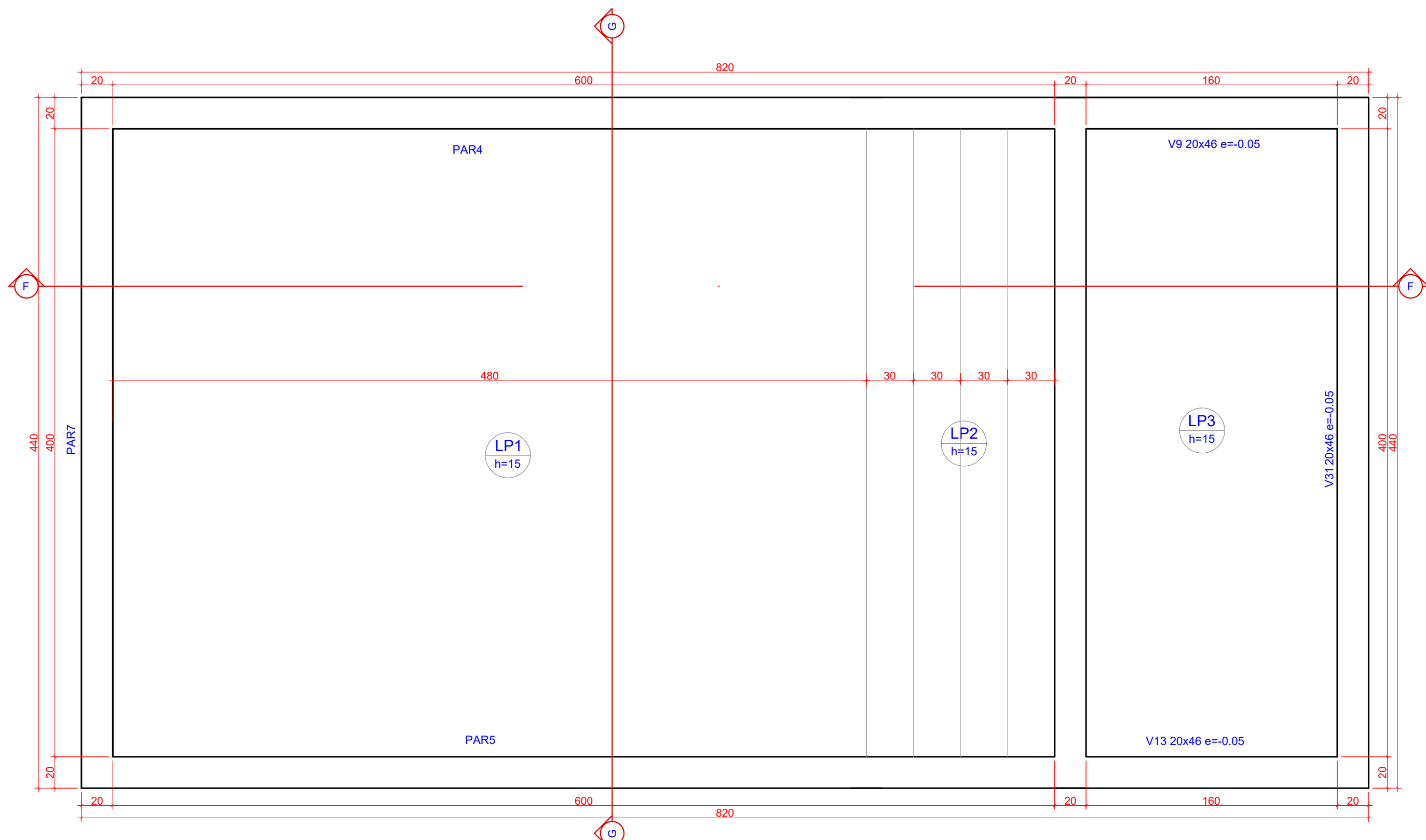
1 PLANTA DE FORMAS: PLANTA BAIXA - PISCINA
