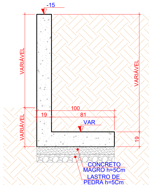
3 PLANTA DE FORMAS - DETALHE MURO M3 ESCALA 1:25
