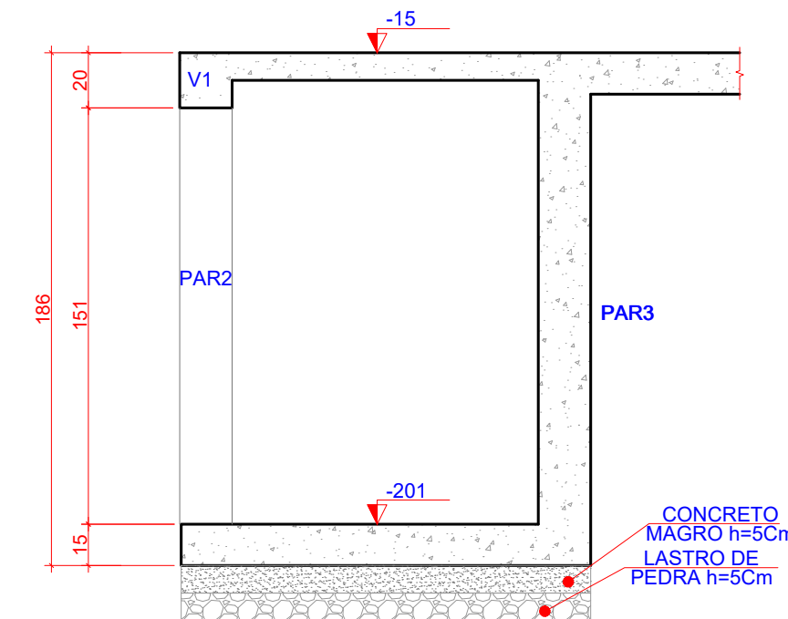
2 PLANTA DE FORMAS: CORTE H-H
