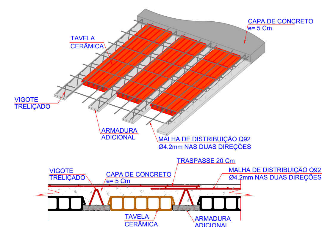
2 DETALHE 01/02 LAJE PRÉ-FABRICADA - TRELIÇADA ESCALA 1:20
