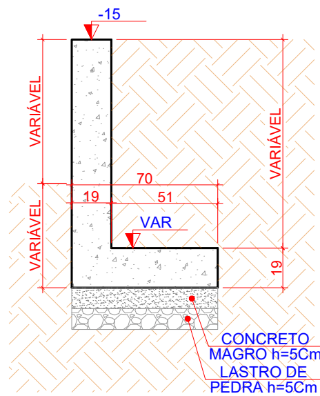
1 PLANTA DE FORMAS - DETALHE MURO M1 ESCALA 1:25
