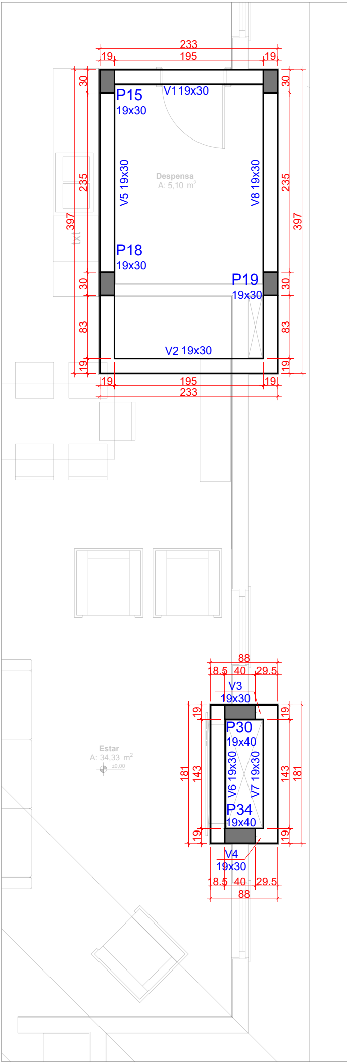
2 PLANTA DE FORMAS - TOPO RESERVATÓRIO (NÍVEL 5.80) ESCALA 1:50
