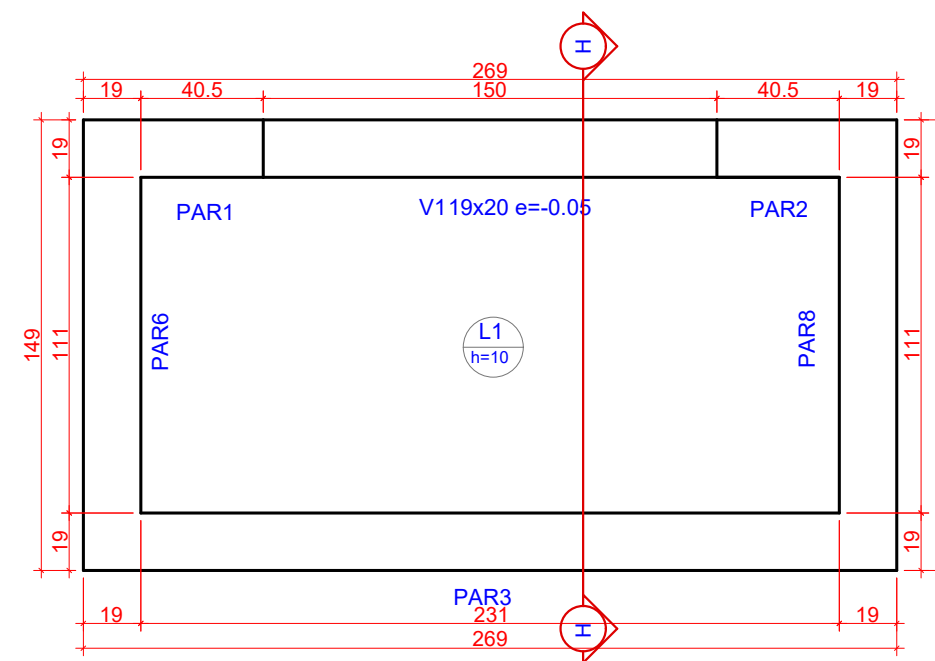
4 PLANTA DE FORMAS: PLANTA BAIXA CASA DE MÁQUINAS
