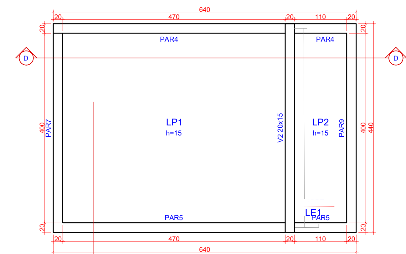
1 PLANTA DE FORMAS - FUNDO PISCINA (NÍVEL -1.36) ESCALA 1:50
