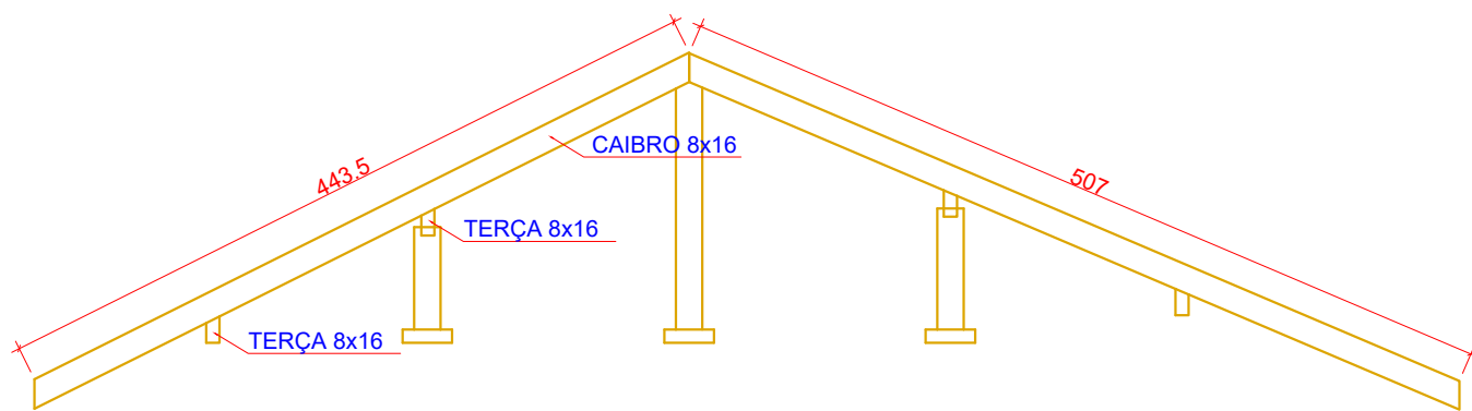
1 CORTE B-B - COBERTURA MADEIRA ESCALA 1:50
