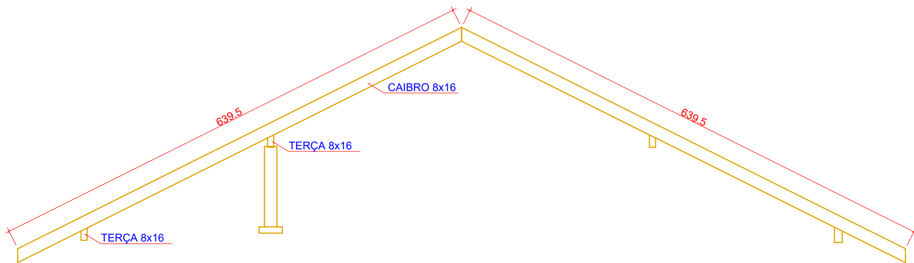
1 CORTE A-A - COBERTURA MADEIRA ESCALA 1:50
