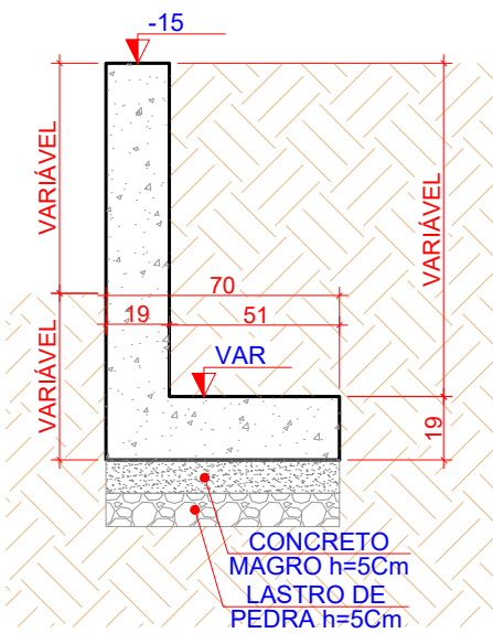
2 PLANTA DE FORMAS - DETALHE MURO M2 ESCALA 1:25
