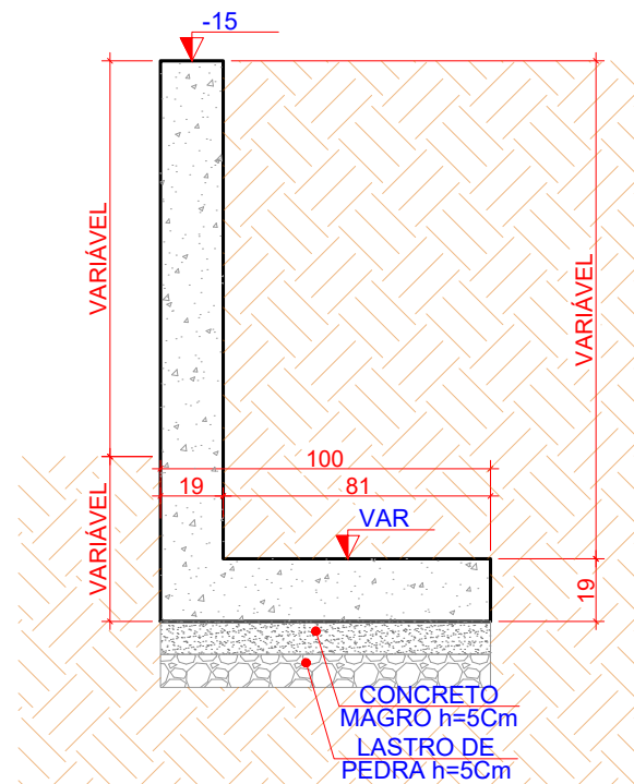
4 PLANTA DE FORMAS - DETALHE MURO M4 ESCALA 1:25
