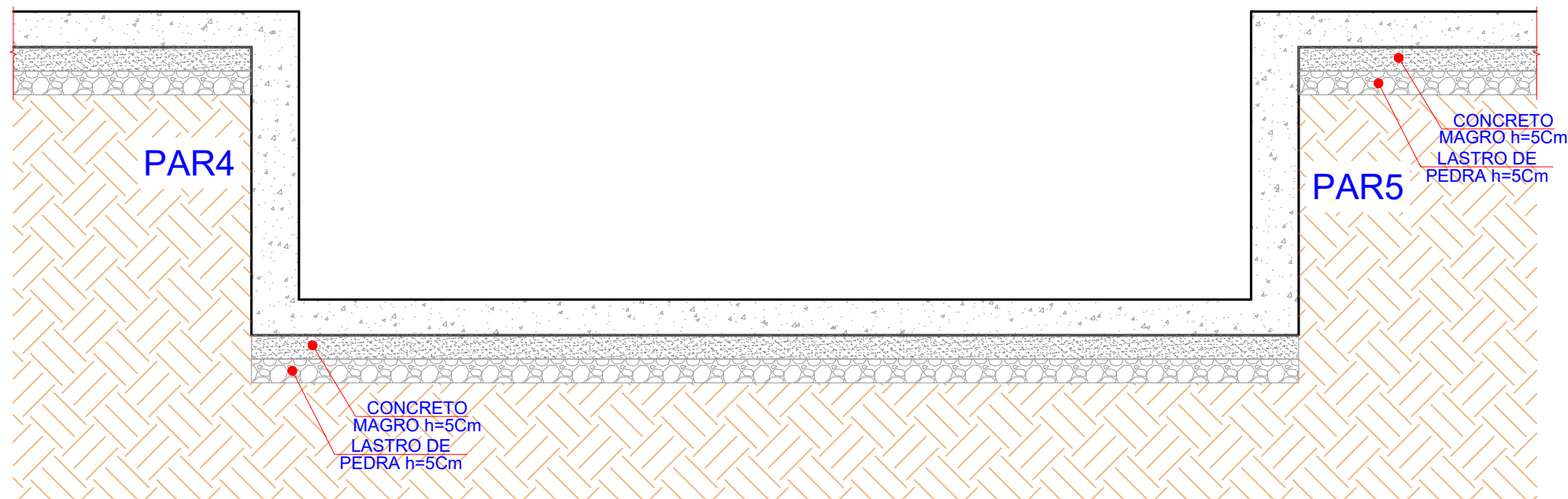
3 PLANTA DE FORMAS: CORTE G-G
