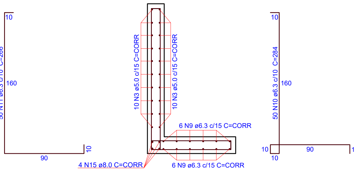
7 PLANTA DE ARMADURAS - DETALHE MURO M3 ESCALA 1:25
