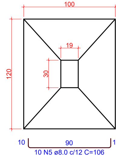
S10=S13=S28=S32 PLANTA ESC 1:25
