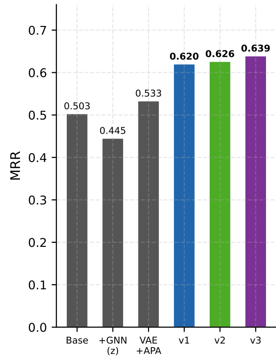
(b) MRR
