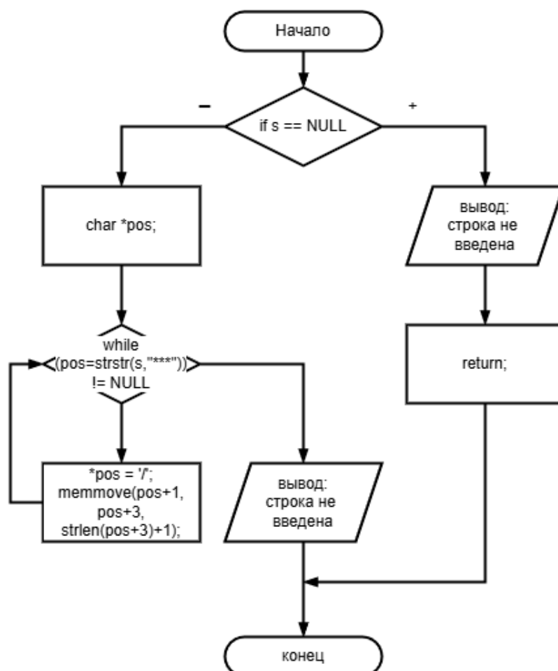
Рисунок 1.7 – Структурная схема функции replaceStars(s) для языка C
