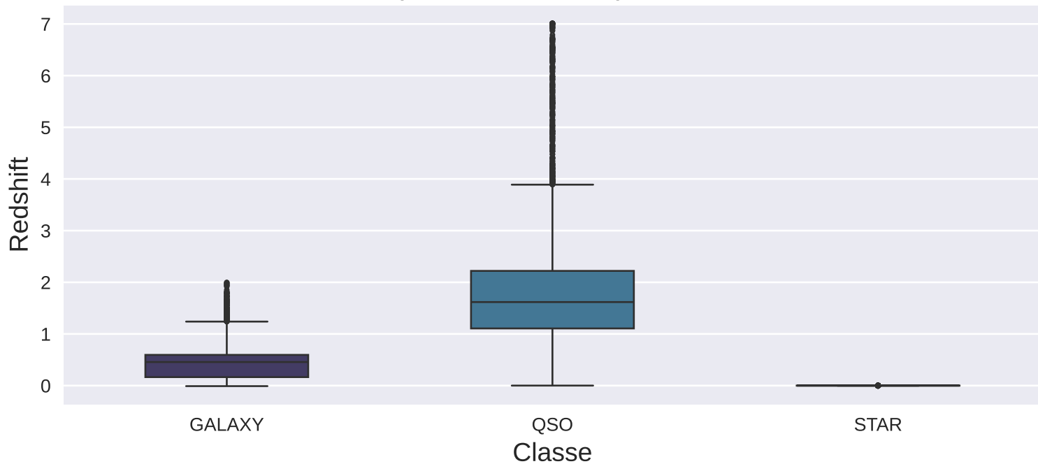
Boxplot de Redshift por Classe
