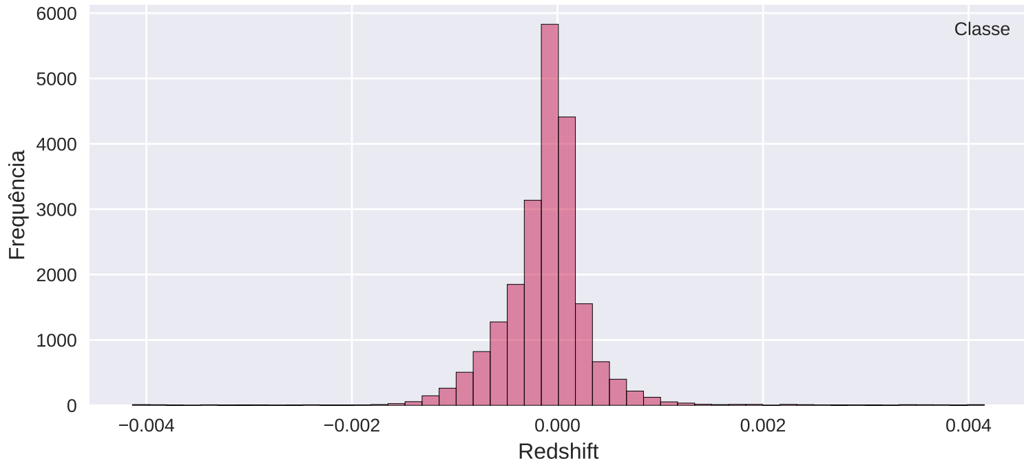
Distribuição do Redshift (Estrelas)
