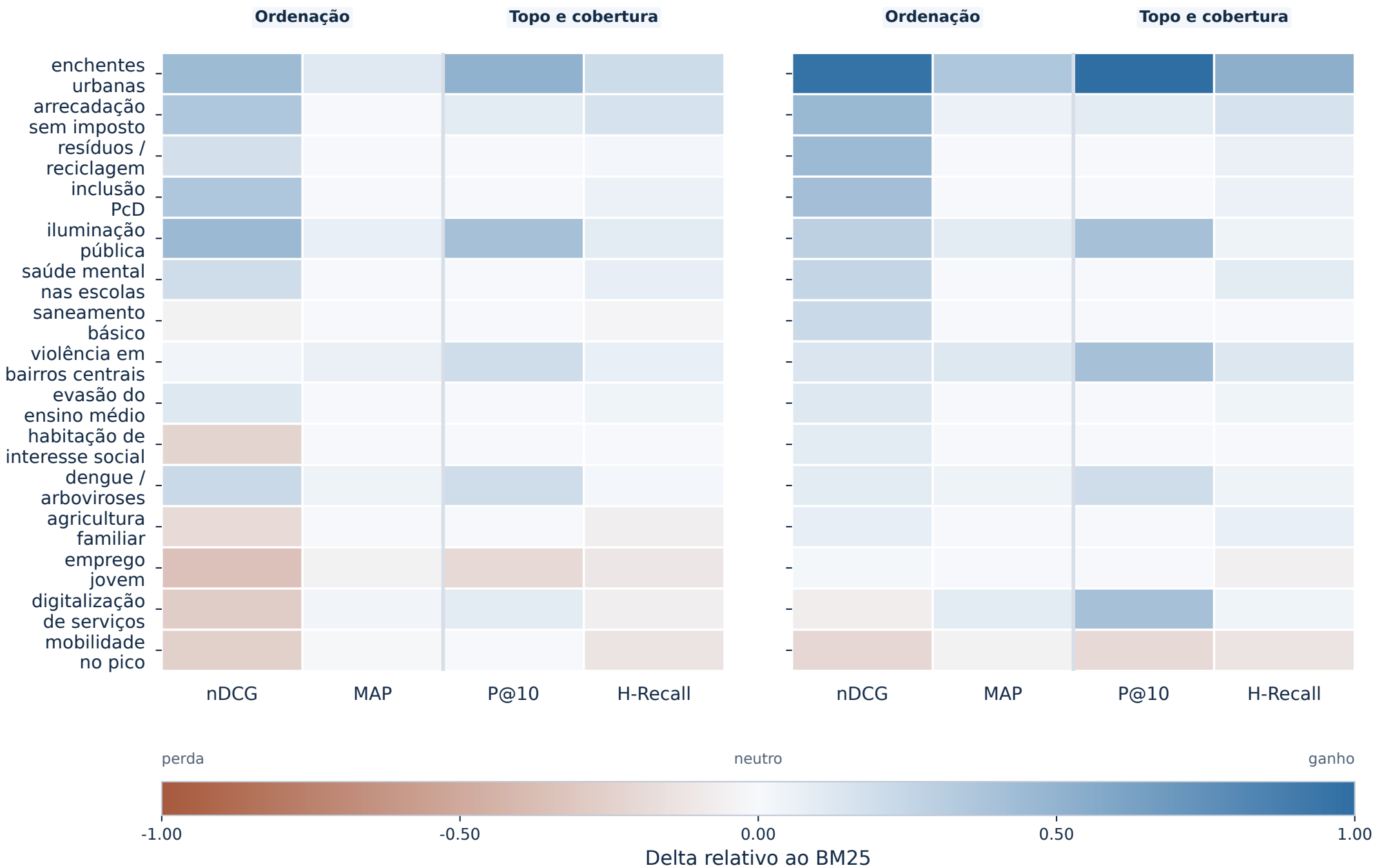
Ações - BM25
