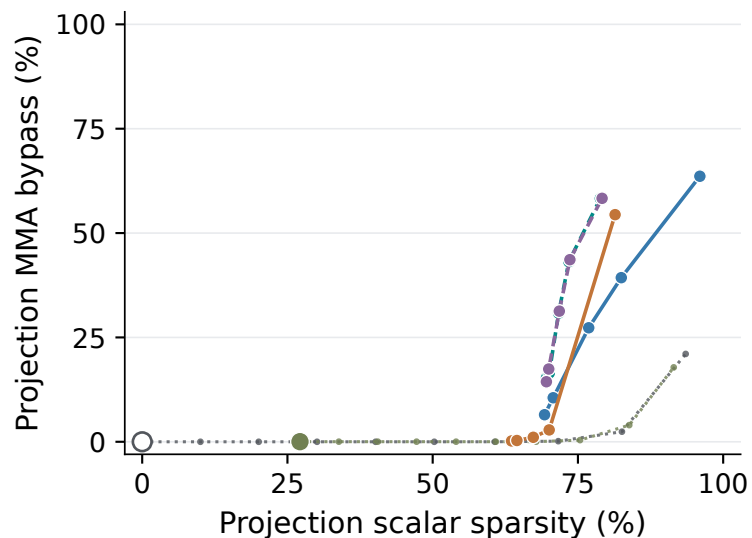
(d) 70M: Sparsity and bypass
