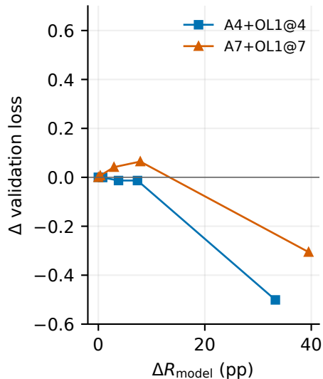
410M
