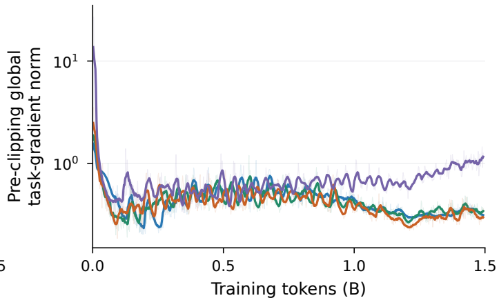
(b) T_0/P_0 gradient norm
