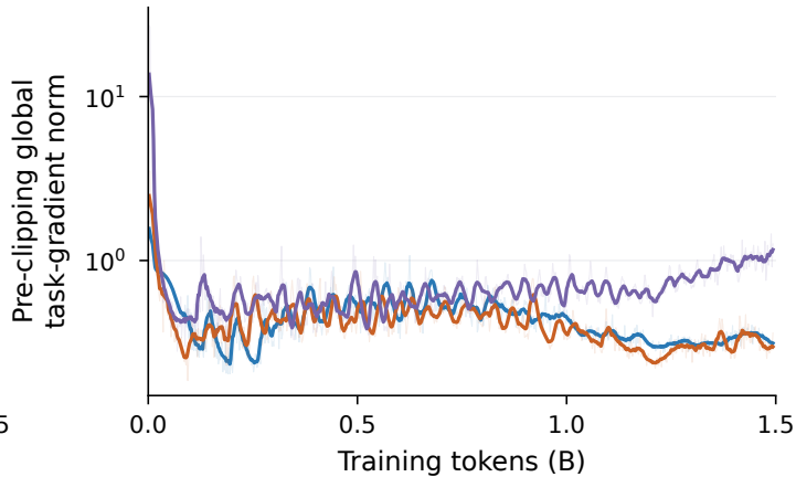
(b) A0 gradient norm
