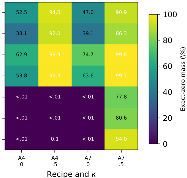
Pythia-410M
