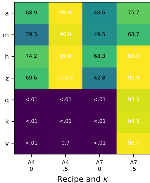
Pythia-14M
