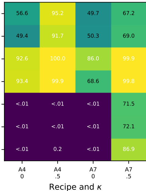
Pythia-70M
