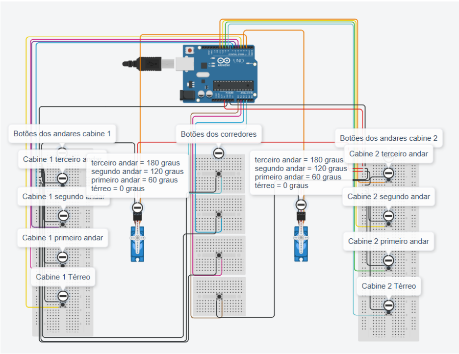
Figura 1 – Montagem Tinkercad
