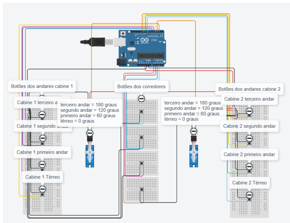
Figura 1 – Montagem Tinkercad
