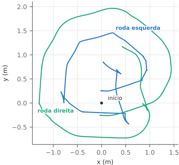
Trajetoória das rodas (odometria de encoders)
