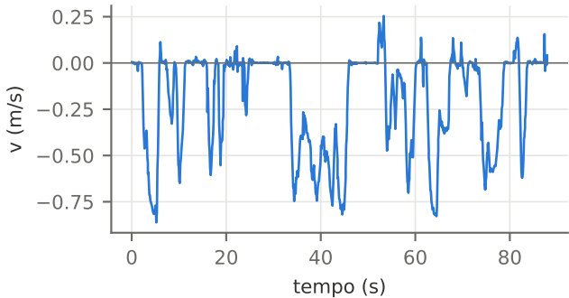
Velocidade linear do robô (derivada das rodas)
