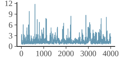
mu_Psi
