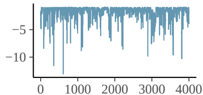
mu_Delta_minus
