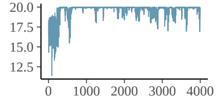
mu_kappa
