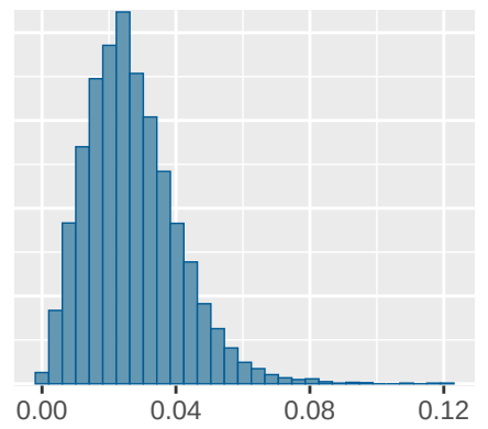
mu_lambda
