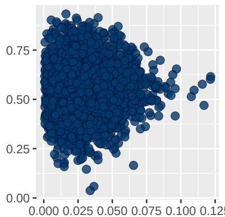
mu_lambda
