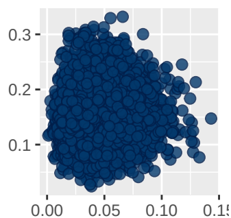
\mu_{\lambda}
