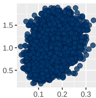
\mu_{\beta}
