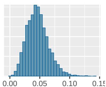
\mu_{\lambda}
