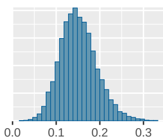
\mu_{\beta}
