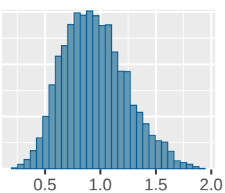
\mu_{\alpha}
