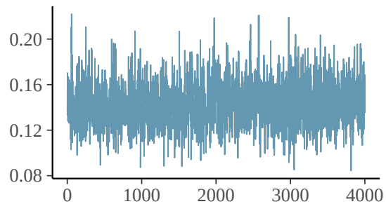
mu_lambda
