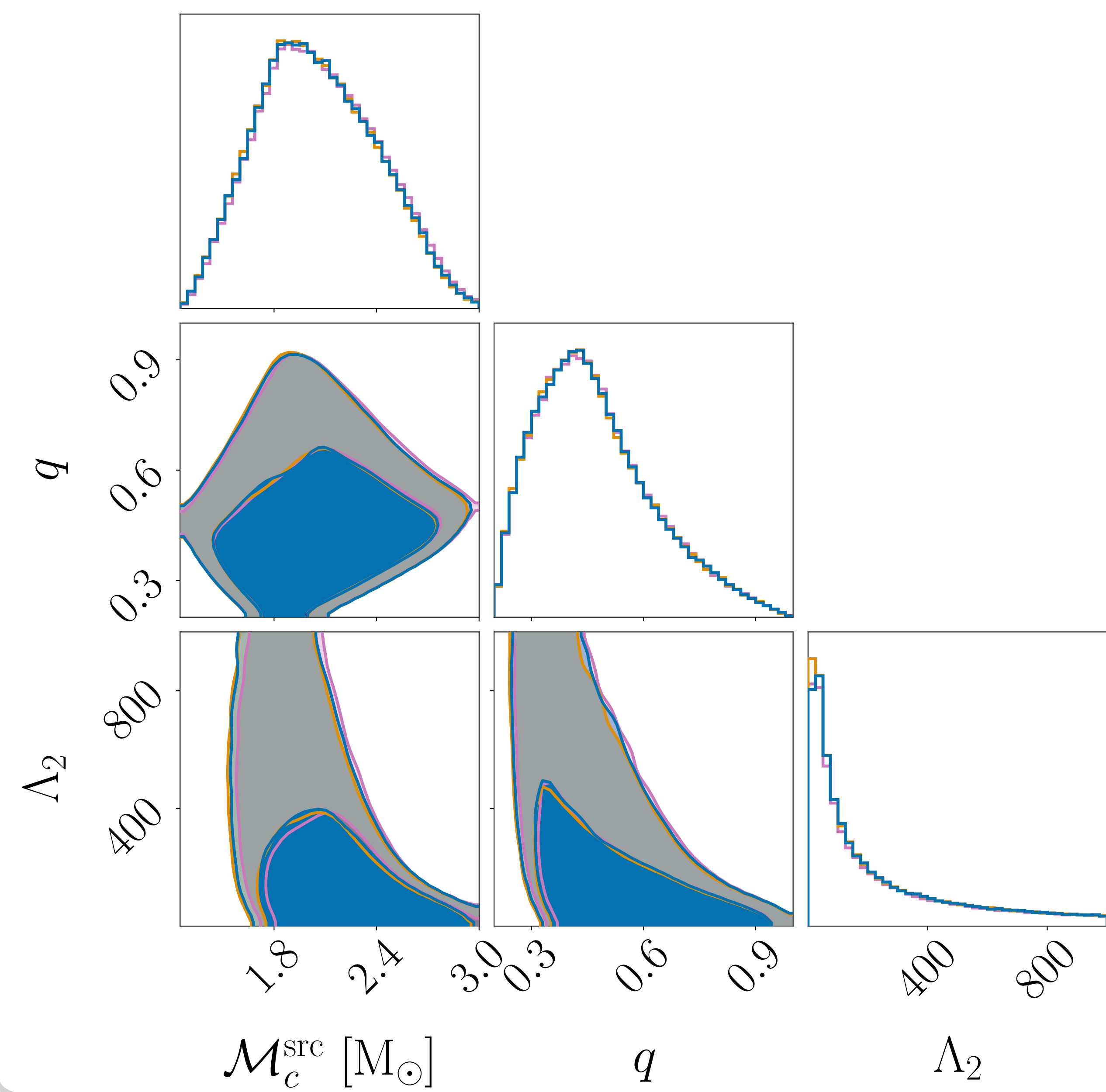
NSBH
