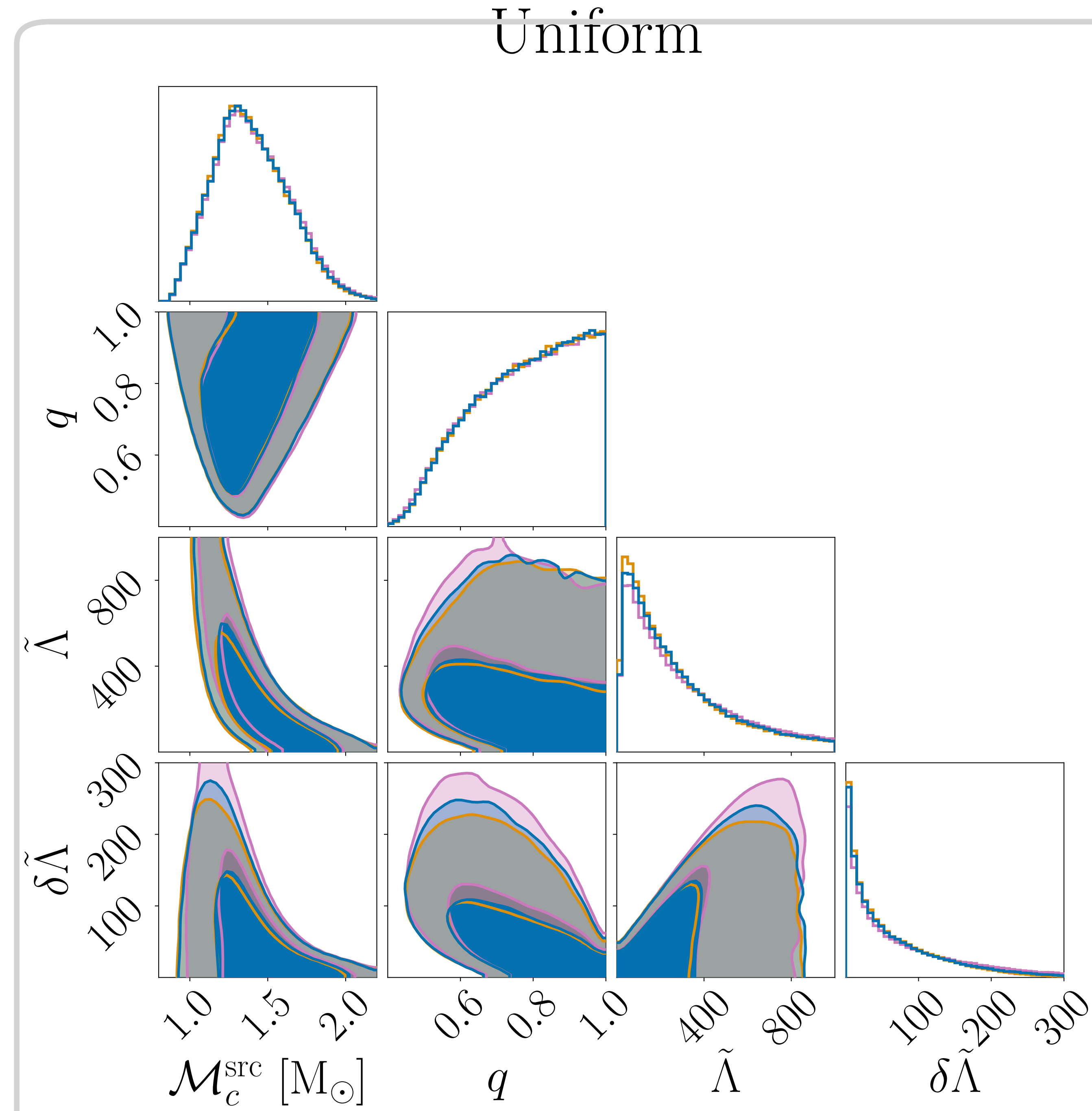
BNS
