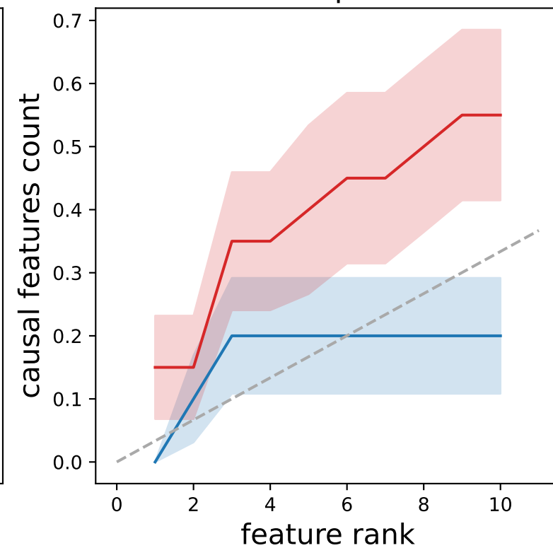
meps
