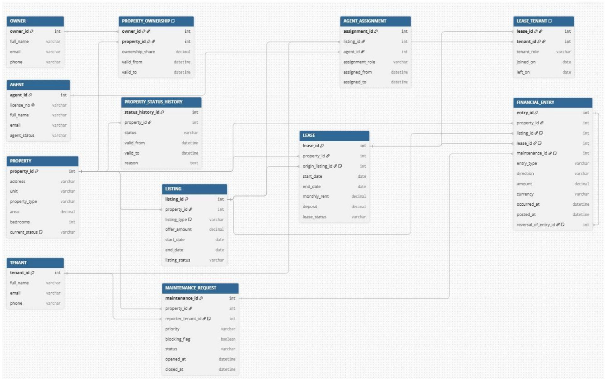
Hình 2. Mô hình ER/EER khái niệm tổng thể theo ký pháp IE Crow's Foot cho Chủ đề 10
