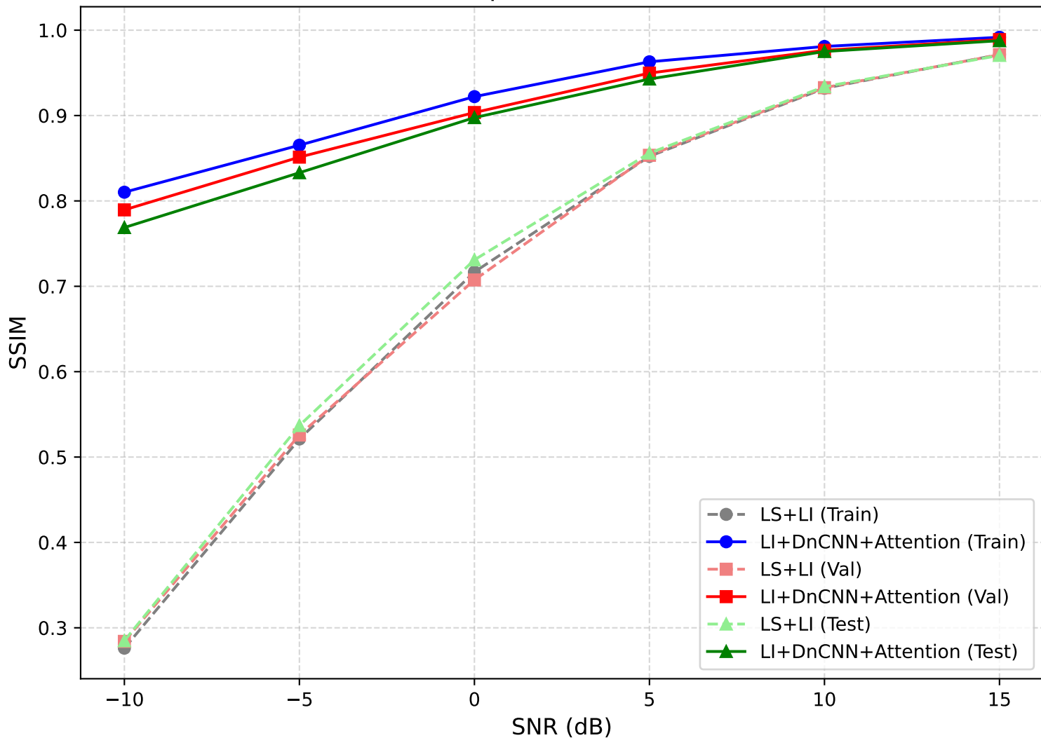
SSIM Comparison over SNR (LI)
