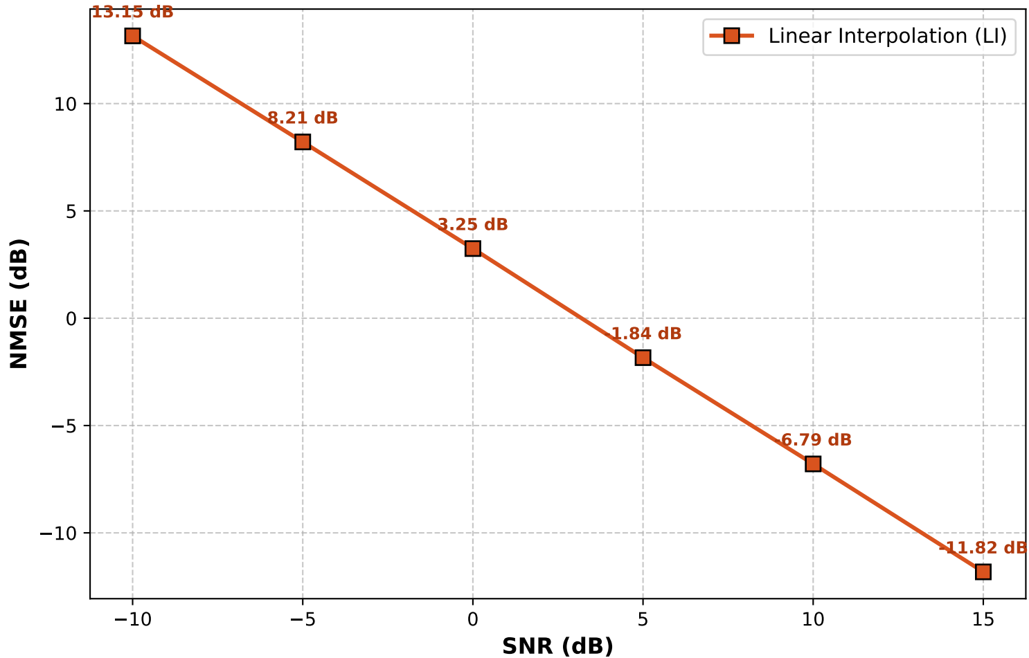
NMSE LI vs. SNR (A100 2.18 GHz 600km 70° 30kHz)
