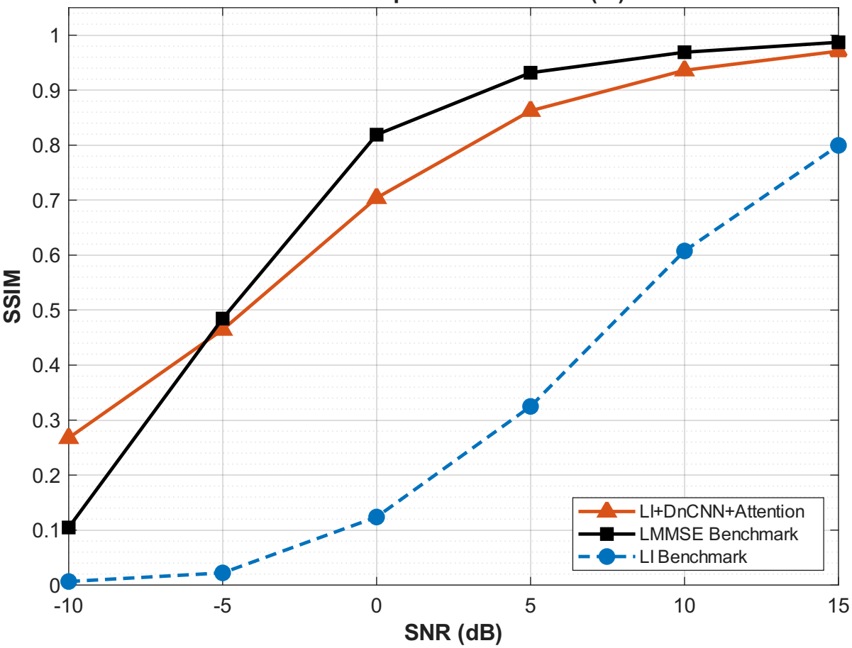
SSIM Comparison over SNR (LI)
