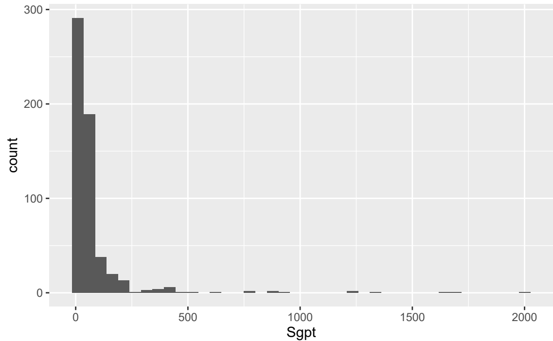
Phân phối Sgpt (trước khi biến đổi log)
