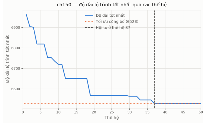
Hình 2.13: Đường hội tụ của GA trên bộ dữ liệu ch150
