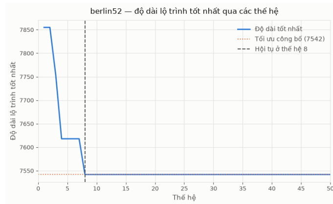
Hình 2.11: Đường hội tụ của GA trên bộ dữ liệu berlin52
