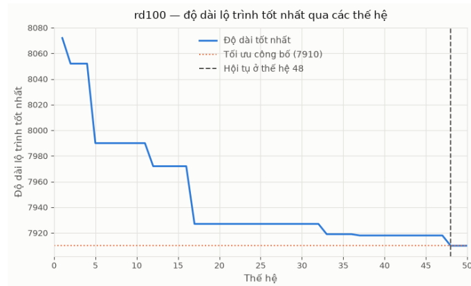
Hình 2.12: Đường hội tụ của GA trên bộ dữ liệu rd100
