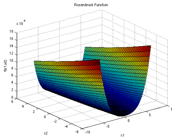
(a) Hàm Rosenbrock trong không gian ba chiều
