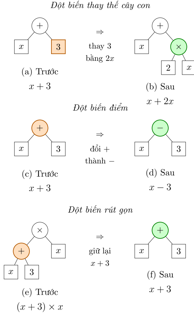
Hình 1.8: Ba toán tử đột biến minh họa trên cây x + 3 (đột biến rút gọn minh họa trên cây lớn hơn (x + 3) \times x ): (a)–(b) đột biến thay thế cây con, (c)–(d) đột biến điểm, (e)–(f) đột biến rút gọn.
