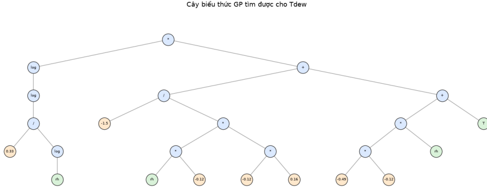
Hình 2.16: Cây biểu thức GP tìm được cho T_{dew}
