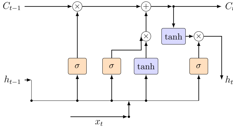
Hình 2: Kiến trúc LSTM cell
