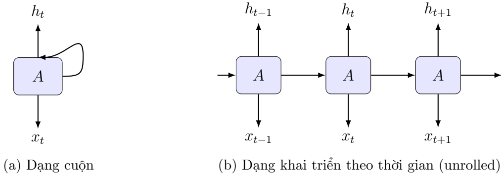
Hình 1: Kiến trúc Recurrent Neural Network (RNN)
