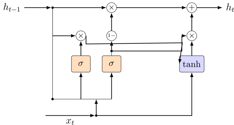
Hình 3: Kiến trúc GRU cell
