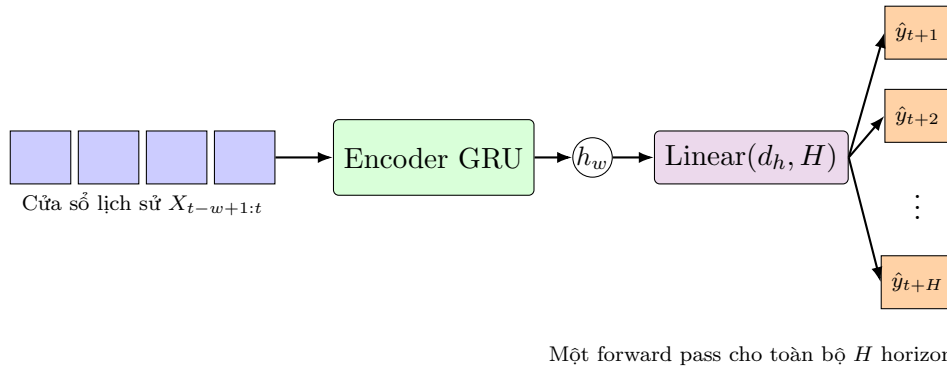
Hình 1.5: Direct Multi-output GRU: Encoder GRU mã hóa cửa sổ lịch sử thành trạng thái ẩn cuối h_w , sau đó lớp Linear sinh đồng thời toàn bộ H giá trị dự báo.
