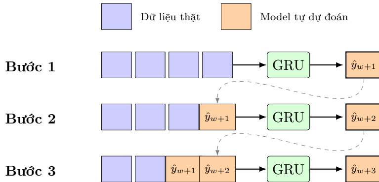
Hình 1.4: Recursive GRU: cửa sổ trượt, phần dự đoán ở bước trước bị đưa ngược vào làm input cho bước sau
