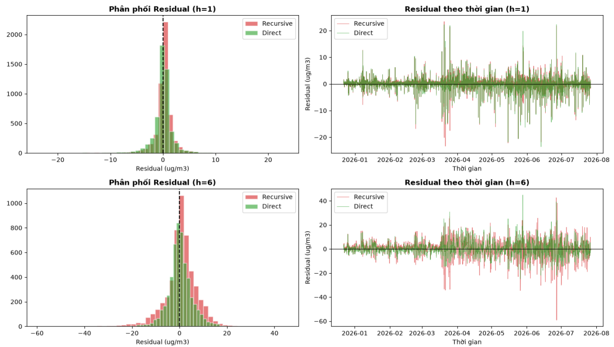
Hình 2.18: Phân phối và diễn biến Residual của Recursive GRU và Direct GRU tại h = 1 và h = 6
