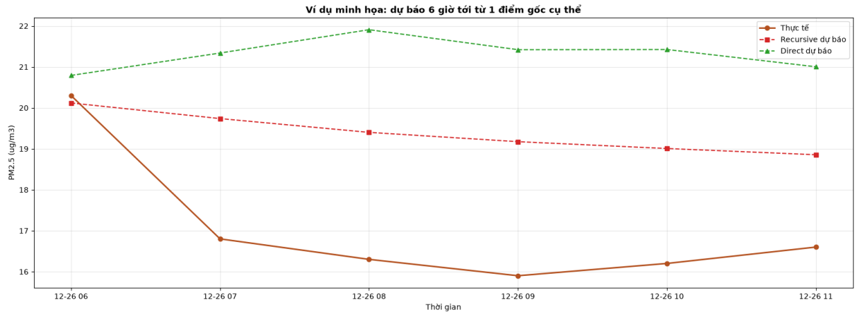
Hình 2.17: Ví dụ minh họa dự báo 6 giờ tới từ một điểm gốc cụ thể trong tập Test
