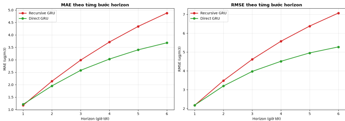
Hình 2.16: MAE và RMSE của Recursive GRU và Direct GRU theo từng bước horizon
