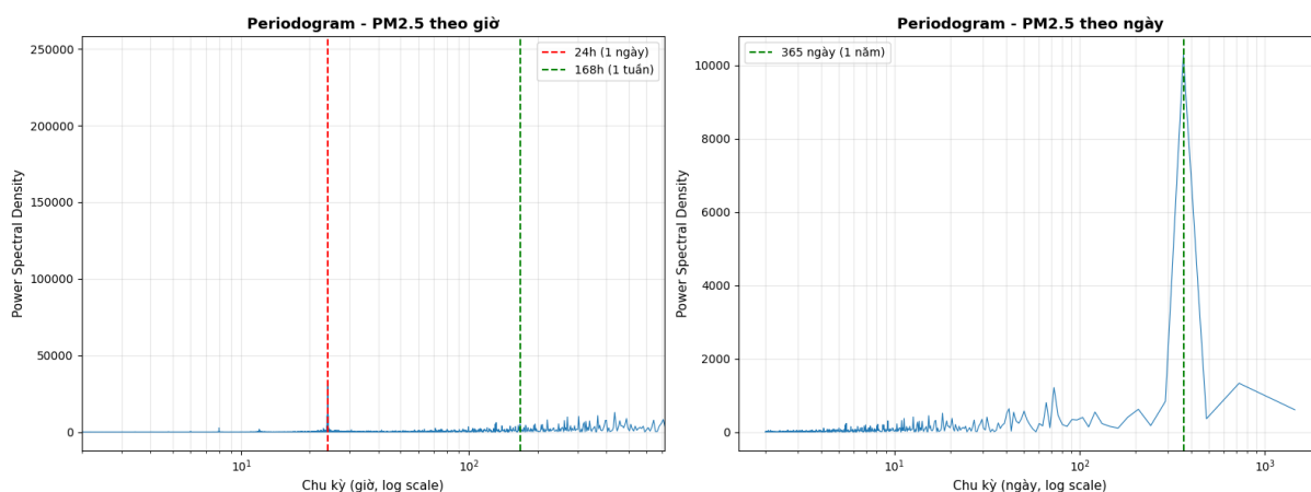
Hình 2.6: Periodogram (FFT) của PM2.5 — xác nhận các chu kỳ chiếm ưu thế
