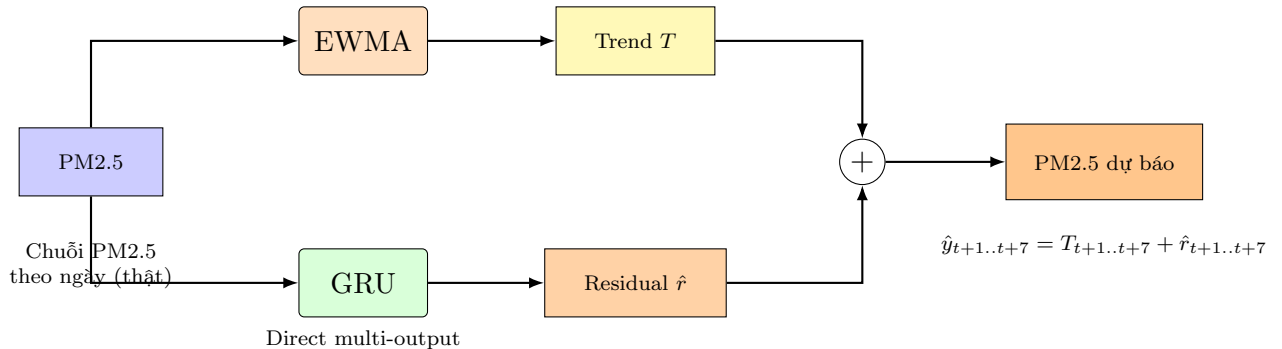
Hình 2.10: Kiến trúc hybrid: EWMA ước lượng Trend, GRU học Residual, cộng lại thành PM2.5 dự báo
