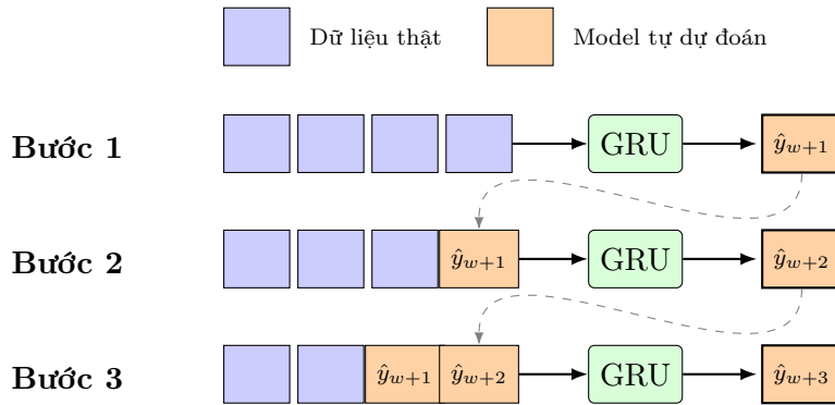
Hình 1.4: Recursive GRU: cửa sổ trượt, phần dự đoán ở bước trước bị đưa ngược vào làm input cho bước sau
