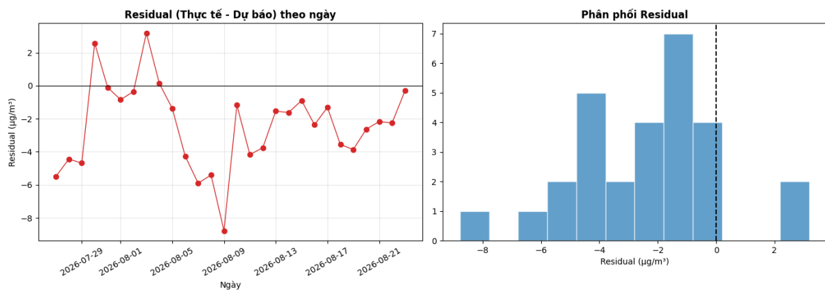
Hình 2.13: Residual (Thực tế – Dự báo) trên tập Test, tổng hợp cả 4 khối walk-forward
