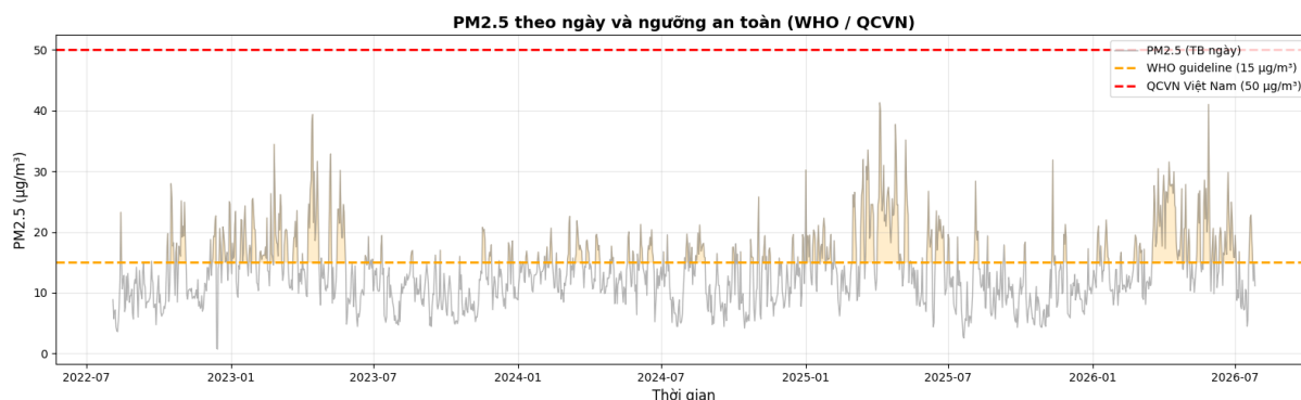
Hình 2.9: PM2.5 trung bình ngày so với ngưỡng khuyến nghị WHO và QCVN Việt Nam
