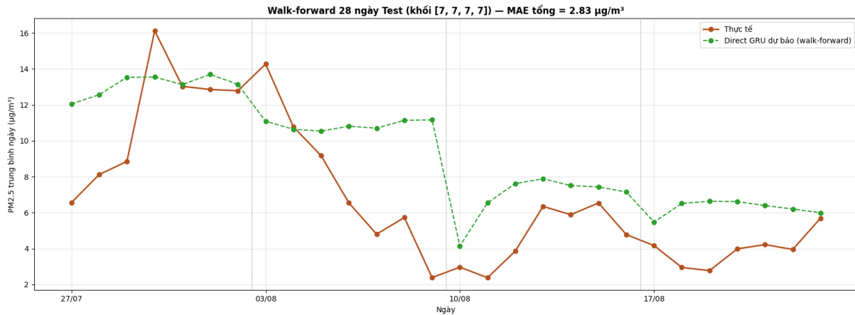
Hình 2.12: PM2.5: Thực tế và Dự báo walk-forward trên tập Test (đường chấm xám đánh dấu ranh giới giữa các khối)
