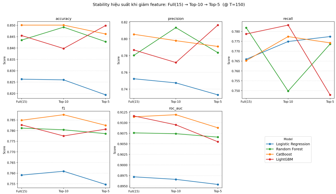
Hình 3.6: Biến động các chỉ số hiệu suất khi giảm số lượng đặc trưng: Full(15) → Top-10 → Top-5, tại mốc 150 ngày.
