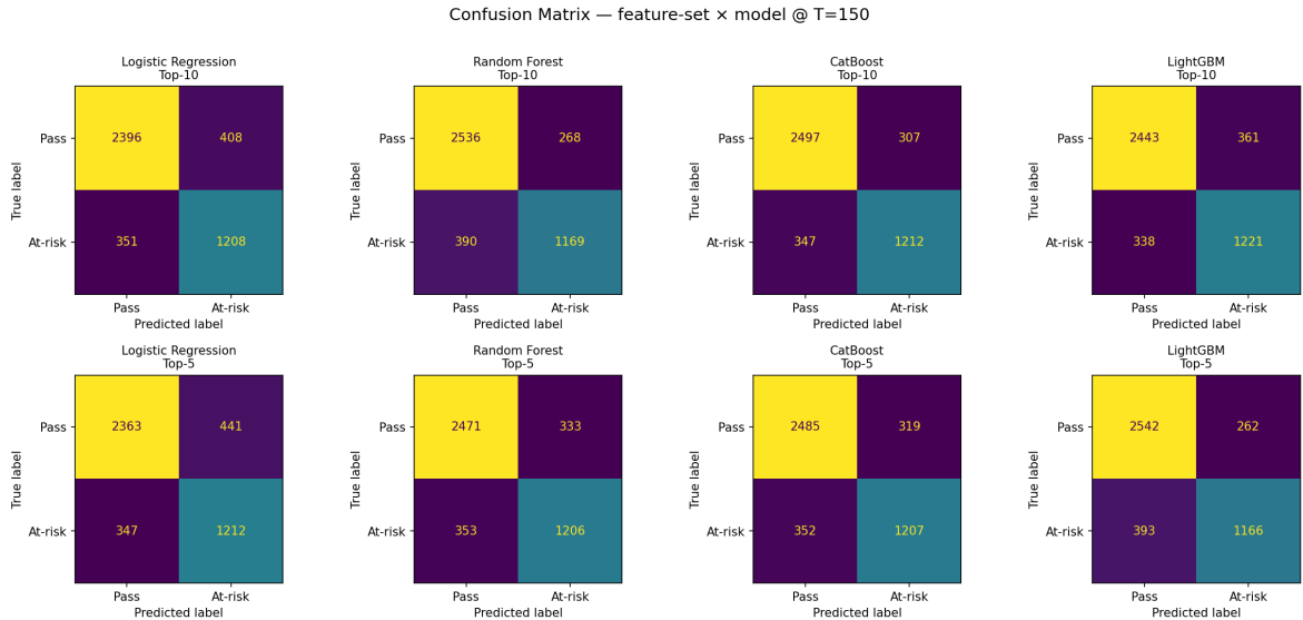
Hình 3.5: Ma trận nhầm lẫn của bốn mô hình trên hai bộ đặc trưng rút gọn Top-10 và Top-5, tại mốc 150 ngày.
