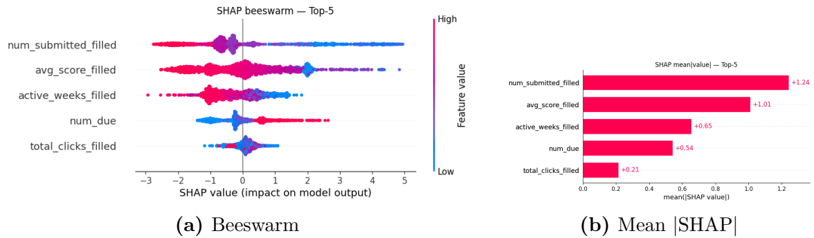
Hình 3.10: Diễn giải SHAP của LightGBM trên bộ đặc trưng Top-5.
