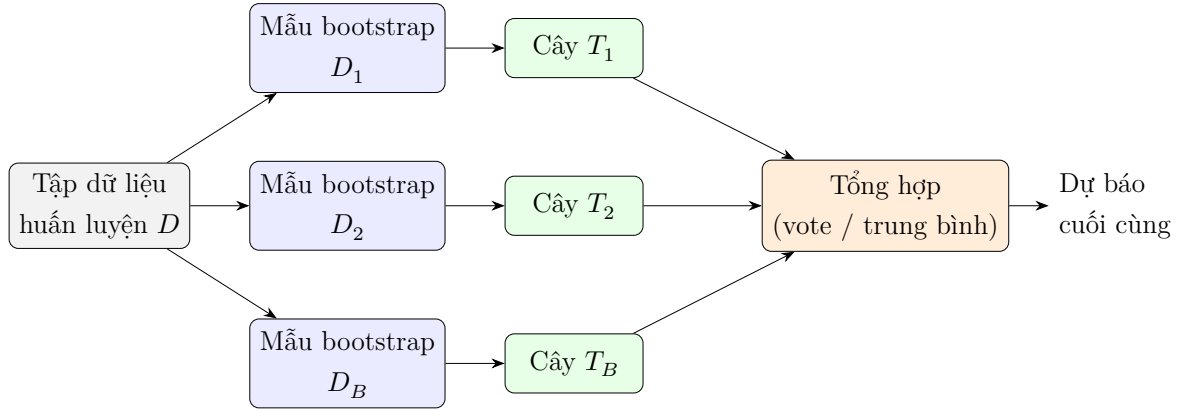
Hình 1.3: Sơ đồ nguyên lý Bagging: B cây được huấn luyện độc lập trên các mẫu bootstrap khác nhau, kết quả được tổng hợp bằng biểu quyết đa số (phân loại) hoặc trung bình (hồi quy).
