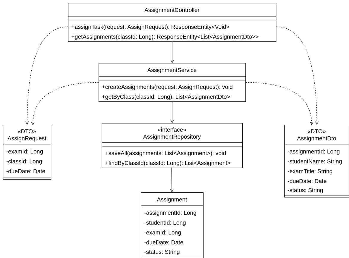
Hình 3.102: 3.2.1 Assign an Assessment Class Diagram – Giao bài tập.
