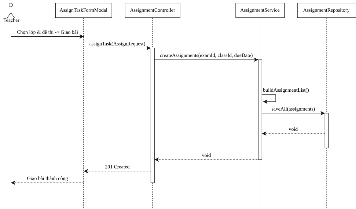
Hình 3.103: 3.2.2 Assign an Assessment Sequence Diagram – Giao bài tập.
