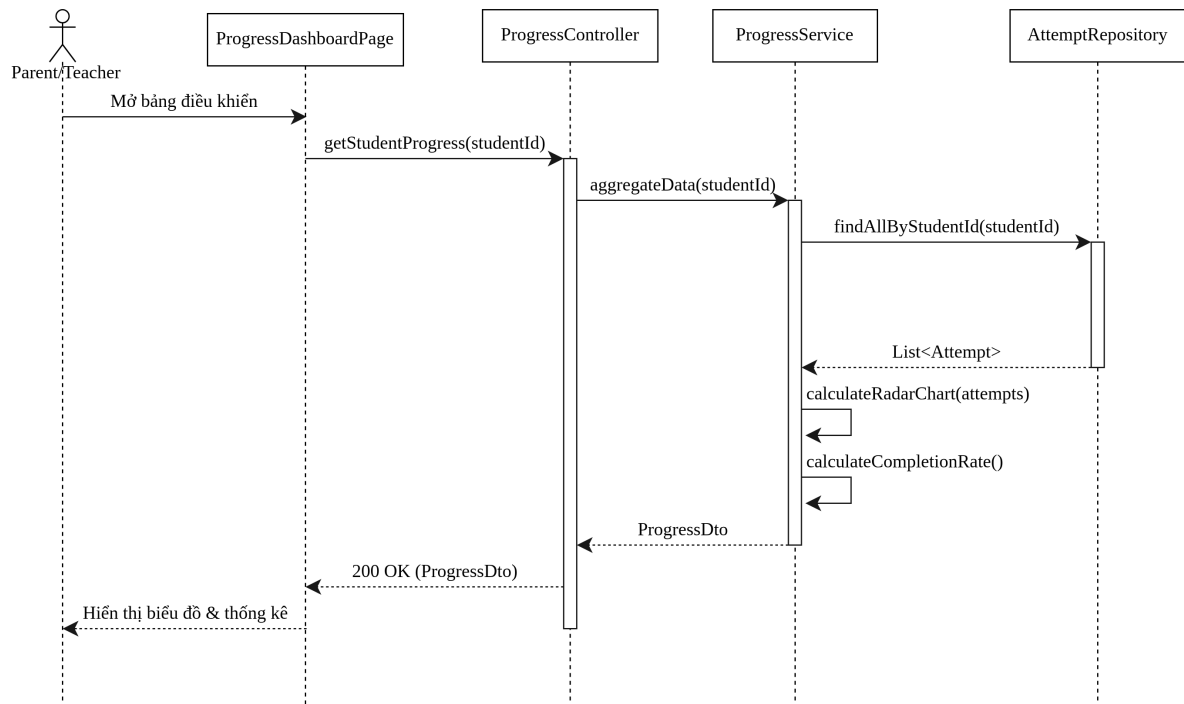
Hình 3.115: 3.8.2 Track Learning Progress Sequence Diagram – Theo dõi tiến độ học tập.
