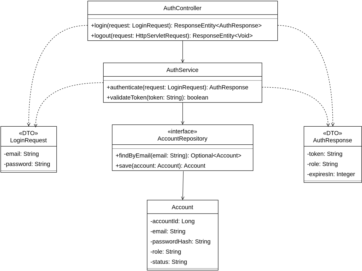
Hình 3.100: 3.1.1 Log in Class Diagram – Xác thực đăng nhập.
