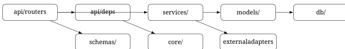
Hình 3.40: Backend package structure baseline.
