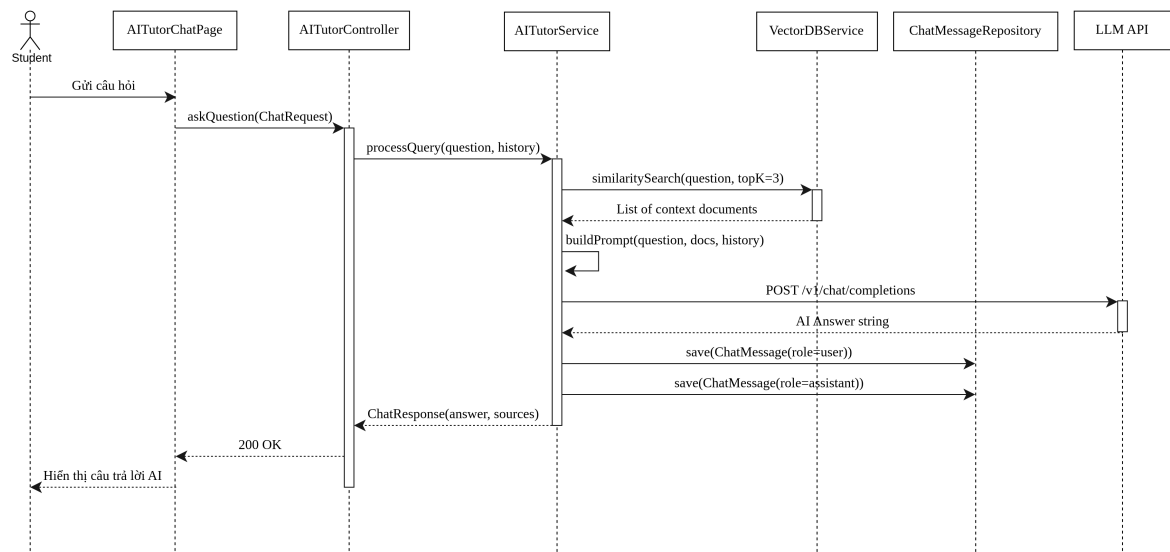
Hình 3.119: 3.10.2 Ask AI Tutor Sequence Diagram – Trợ lý AI.
