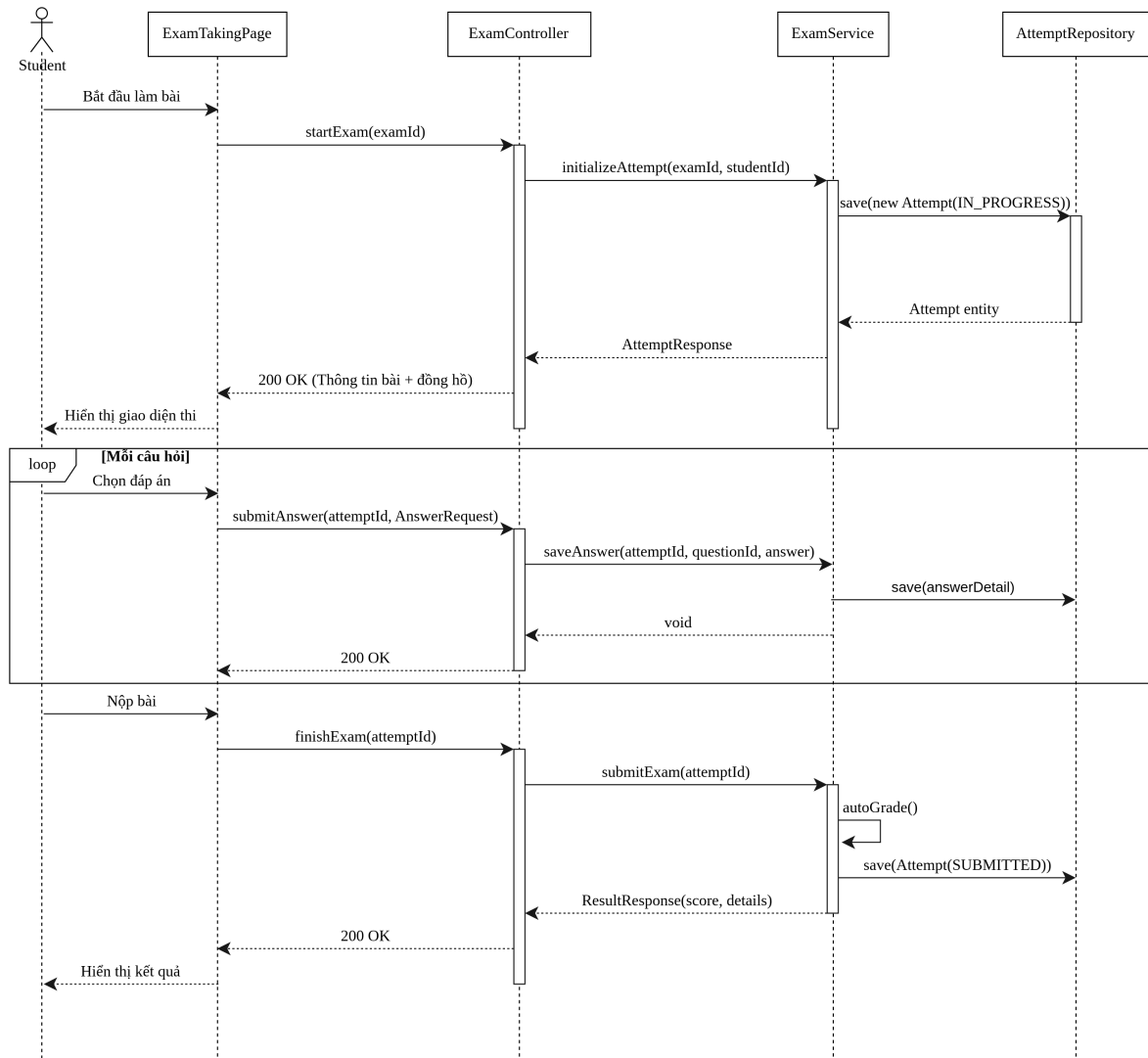
Hình 3.109: 3.5.2 Take Competency Assessment Sequence Diagram – Làm bài thi ĐGNL.
