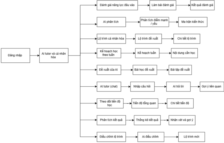
Hình 2: Sơ đồ luồng màn hình AI Tutor Và Cá Nhân Hóa Lộ Trình
