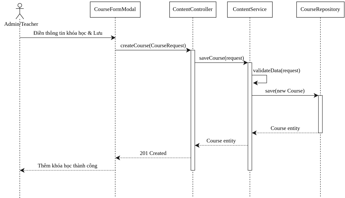
Hình 3.107: 3.4.2 Manage Learning Content Sequence Diagram – Quản lý nội dung học.
