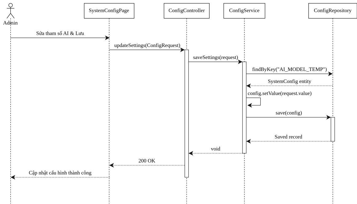
Hình 3.105: 3.3.2 Update System Configuration Sequence Diagram – Cấu hình hệ thống.
