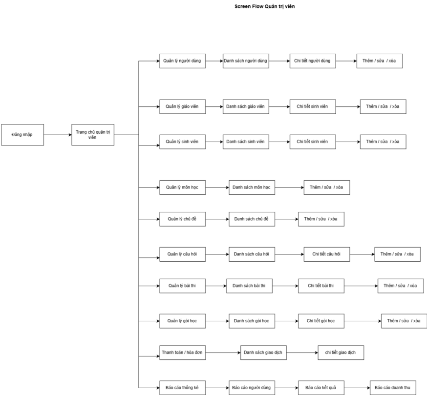
Screen Flow Quản trị viên
