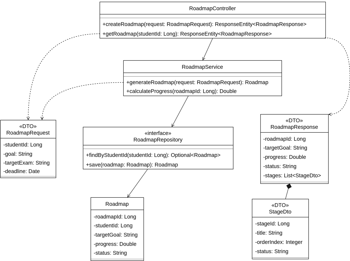
Hình 3.116: 3.9.1 Create Personalized Roadmap Class Diagram – Lộ trình học cá nhân.
