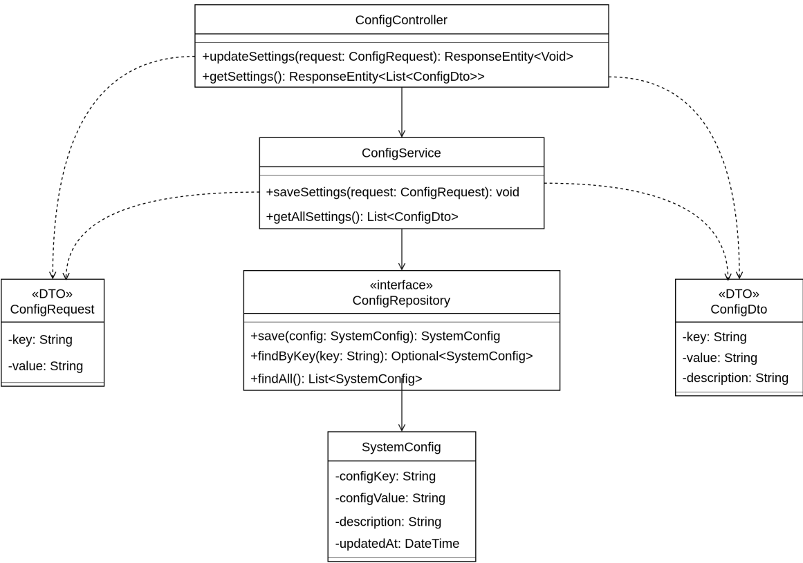
Hình 3.104: 3.3.1 Update System Configuration Class Diagram – Cấu hình hệ thống.
