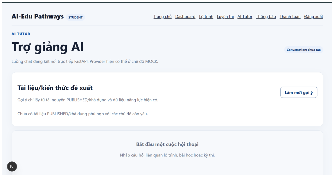
Hình 3.32: Giao diện dùng cho chức năng View Recommended Learning Materials .
