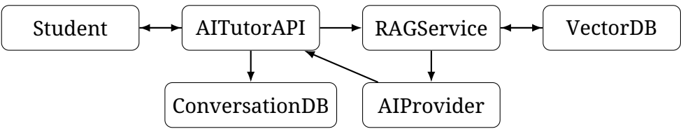
Hình 3.38: AI Tutor + RAG processing flow.
