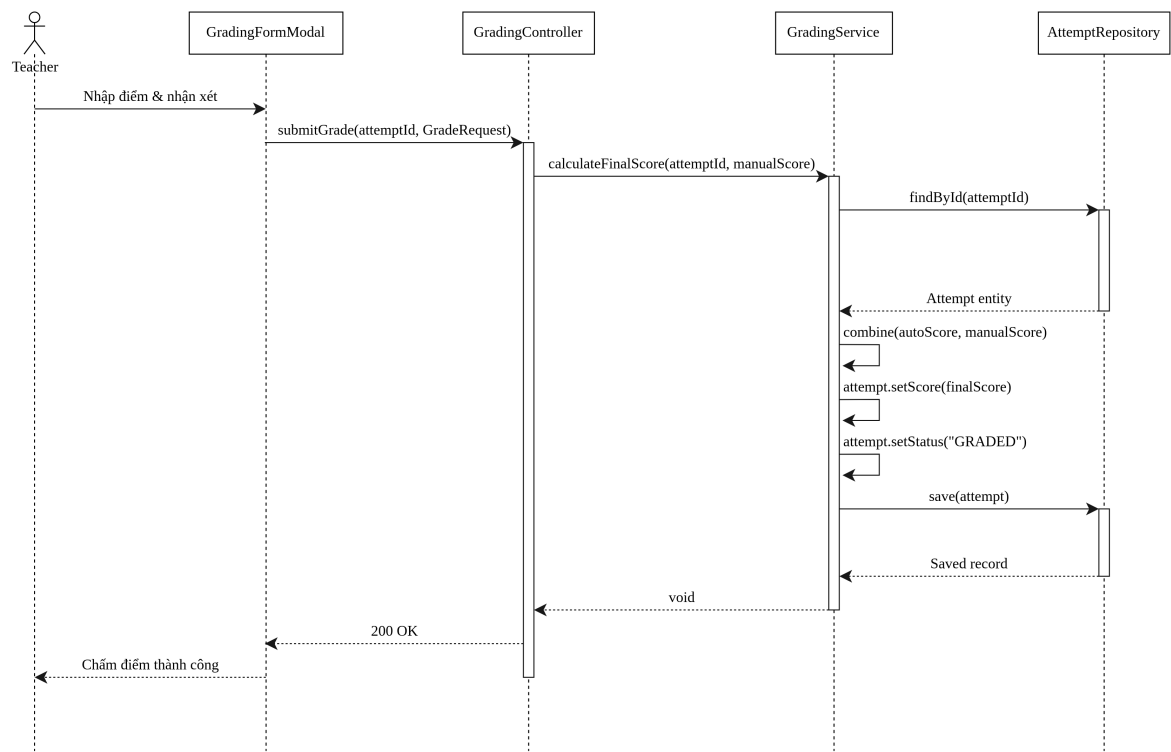
Hình 3.111: 3.6.2 Grade Student Submission Sequence Diagram – Giáo viên chấm điểm.
