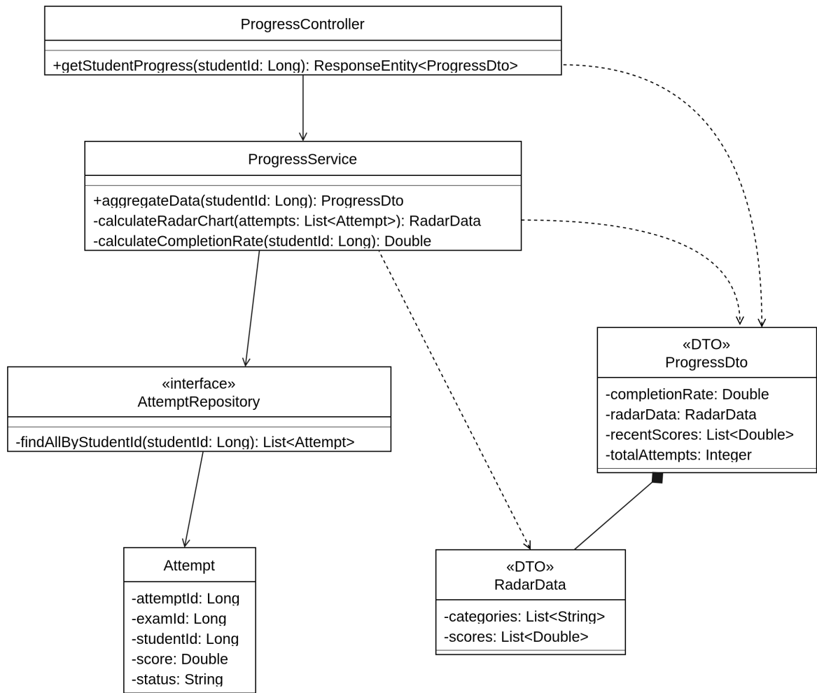
Hình 3.114: 3.8.1 Track Learning Progress Class Diagram – Theo dõi tiến độ học tập.
