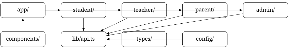
Hình 3.39: Web App package structure baseline.
