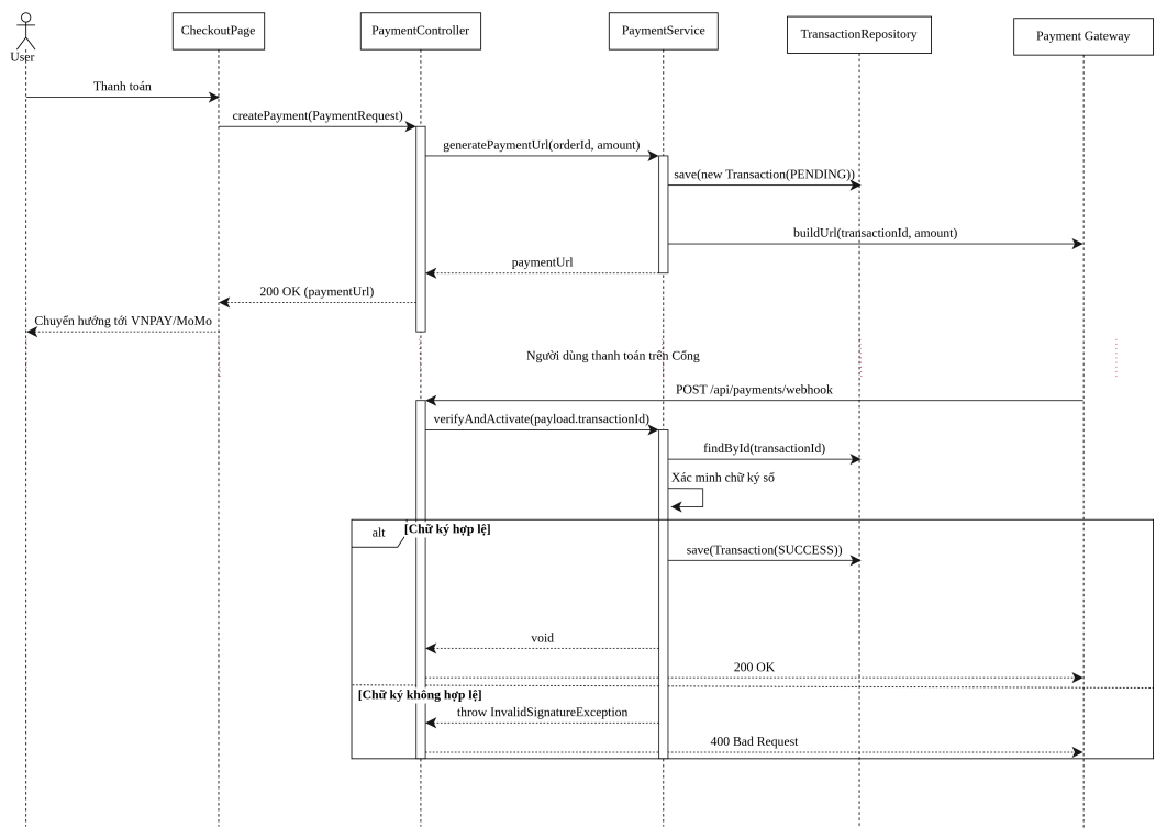
Hình 3.113: 3.7.2 Process Online Payment Sequence Diagram – Thanh toán trực tuyến.
