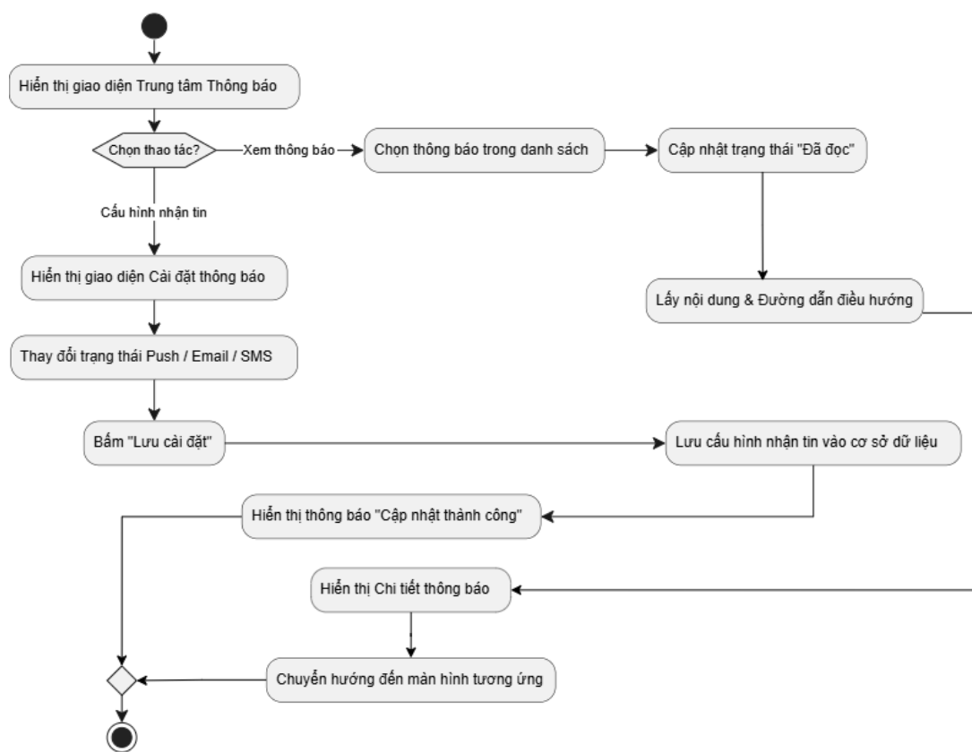
10: Sơ đồ Quản lý Thông báo & Nhắc nhở
