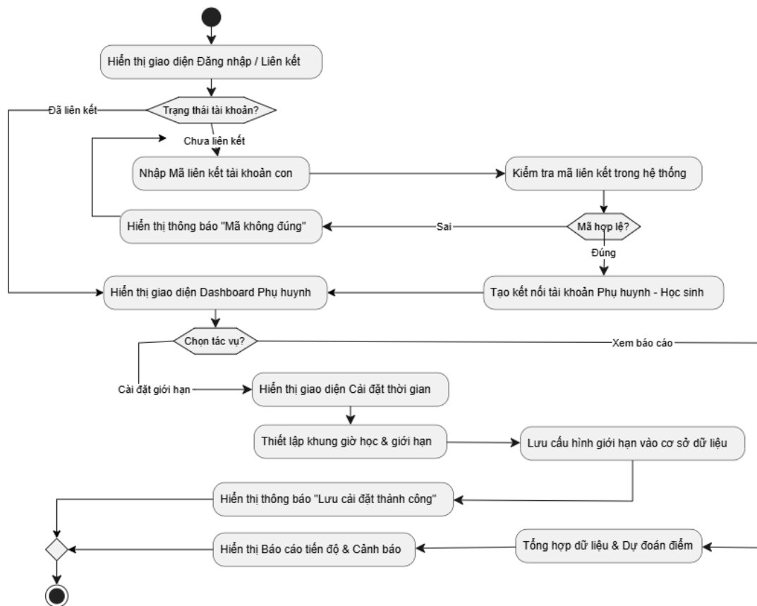
Hình 1.1: Sơ đồ luồng màn hình hệ thống - Phụ huynh
