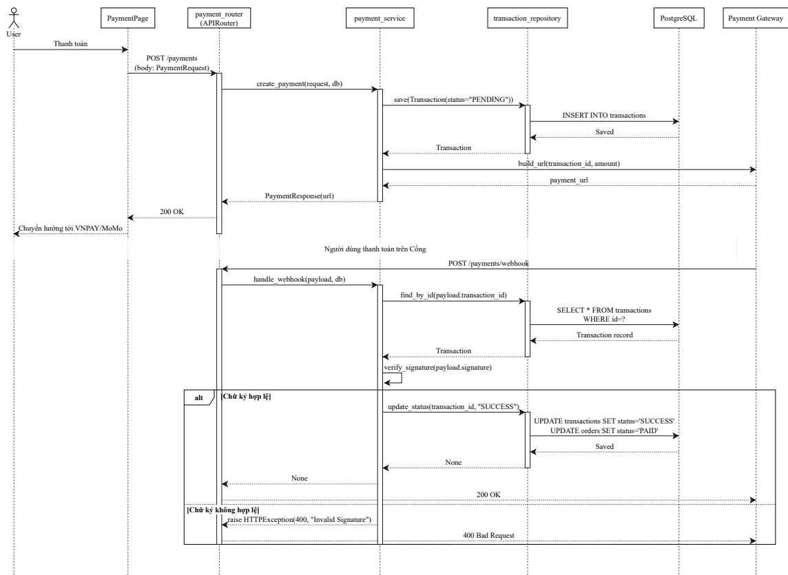
Hình 3.55: 3.7.2 Process Online Payment Sequence Diagram – Thanh toán trực tuyến.
