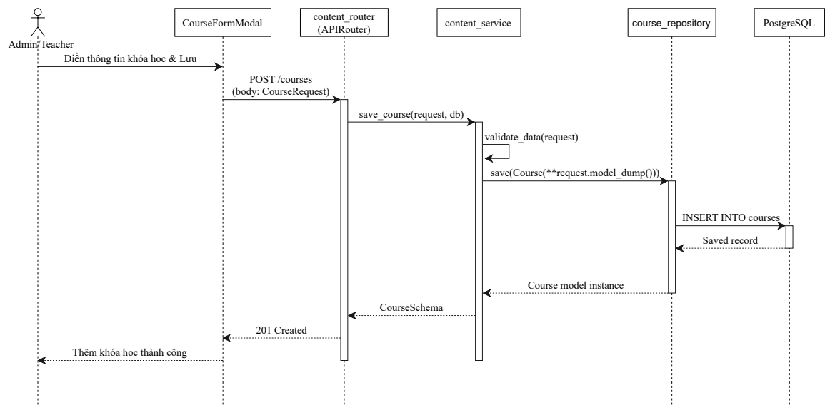
Hình 3.49: 3.4.2 Manage Learning Content Sequence Diagram – Quản lý nội dung học.
