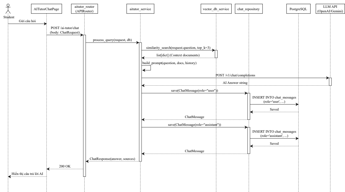
Hình 3.61: 3.10.2 Ask AI Tutor Sequence Diagram – Trợ lý AI.
