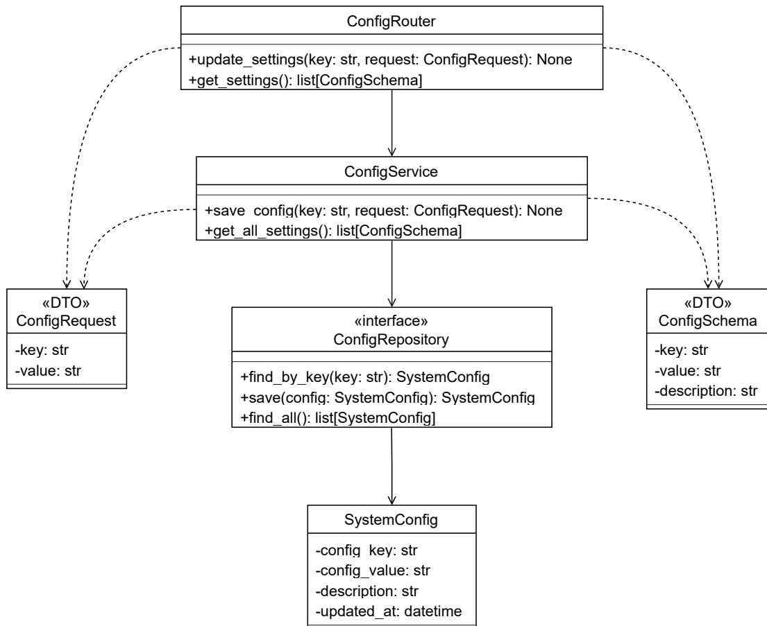
Hình 3.46: 3.3.1 Update System Configuration Class Diagram – Cấu hình hệ thống.
