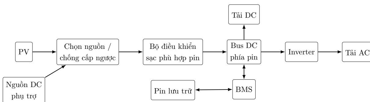
Hình 6.1: Sơ đồ khối luồng năng lượng của hệ thống.
