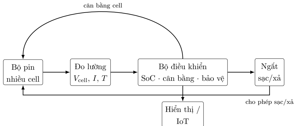
Hình 3.1: Sơ đồ khối chức năng và luồng xử lý của BMS.
