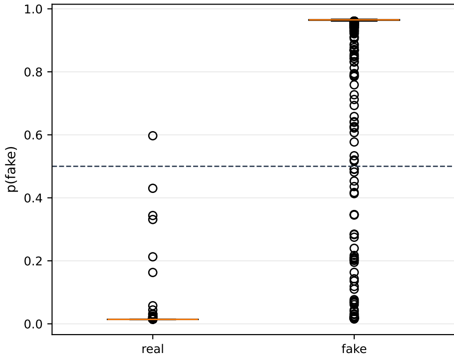
Scores por classe — Conformer
