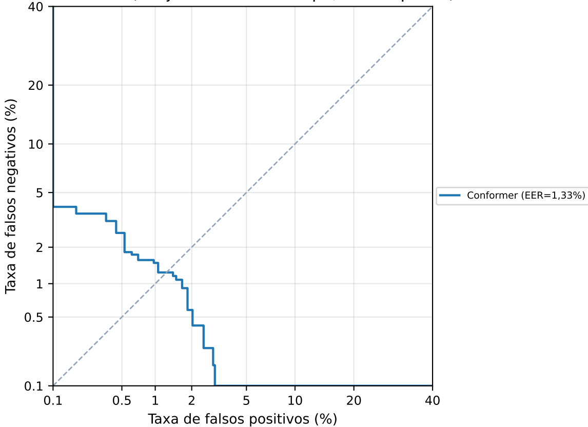
Curvas DET (conjunto de teste limpo, escala probit)
